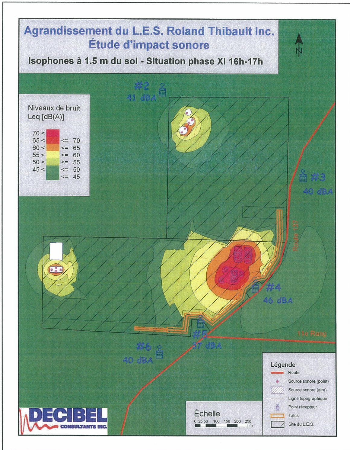
Figure 6 : Isophones générés par les activités d'exploitation de la phase XI et d'aménagement de la phase XII du futur site d'enfouissement du L.E.T. entre 16 h et 17 h
