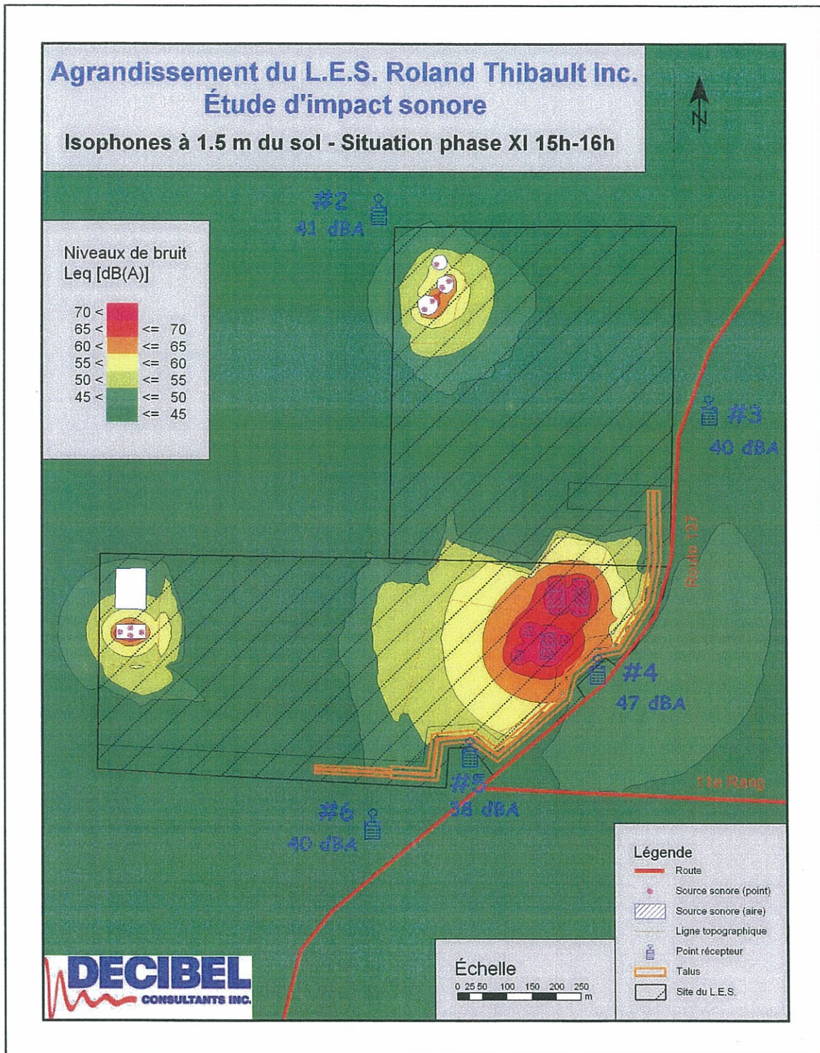
Figure 5 : Isophones générés par les activités d'exploitation de la phase XI et d'aménagement de la phase XII du futur site d'enfouissement du L.E.T. entre 15 h et 16 h
