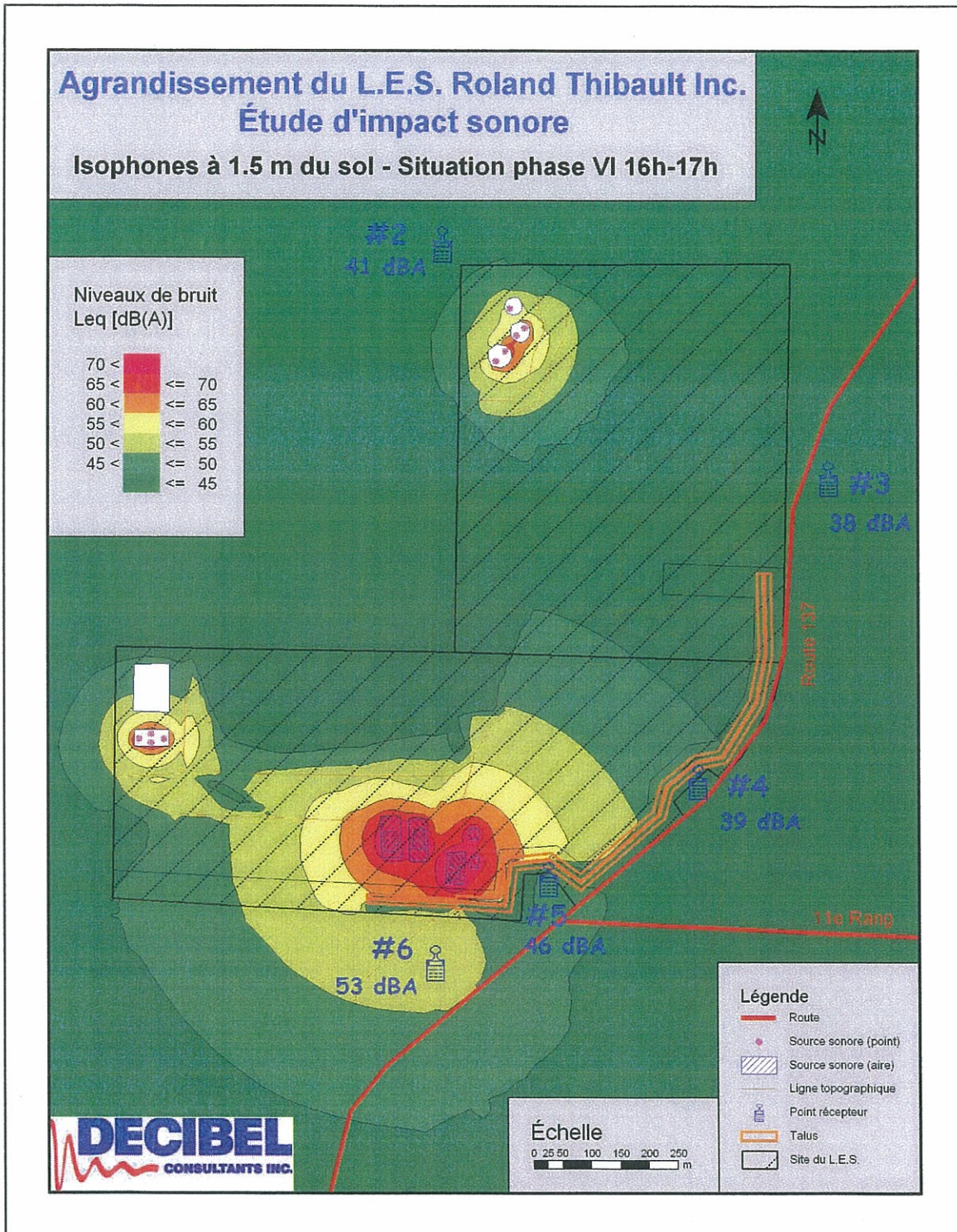
Figure 4 : Isophones générés par les activités d'exploitation de la phase VI et d'aménagement de la phase VII du futur site d'enfouissement technique entre 16 h et 17 h
