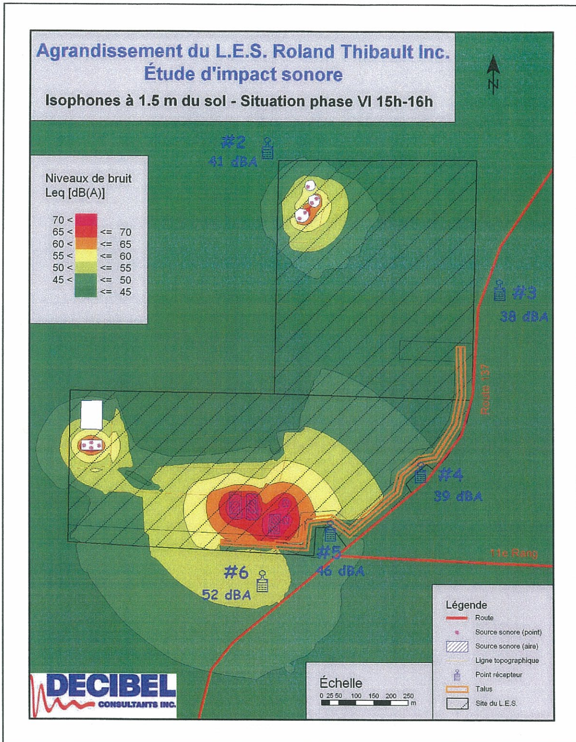
Figure 3 : Isophones générés par les activités d'exploitation de la phase VI et d'aménagement de la phase VII du futur site d'enfouissement technique entre 15 h et 16 h
