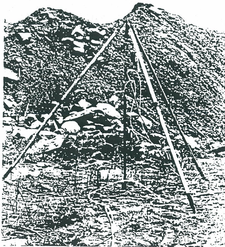
Planche 13. Trépied soutenant les obturateurs et la tubulure
