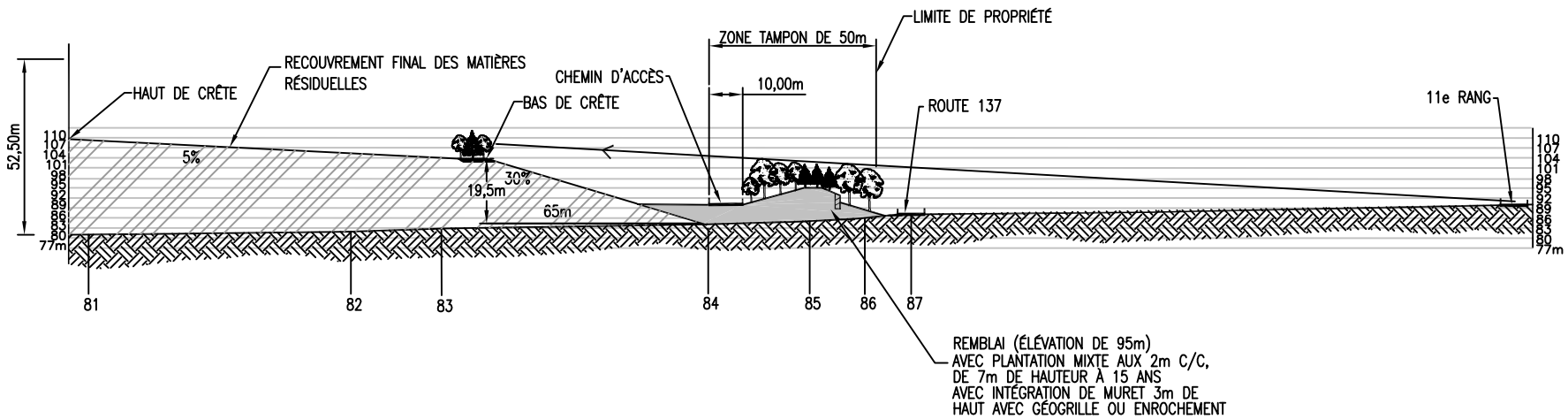
Figure 4.9: Coupe D-D
