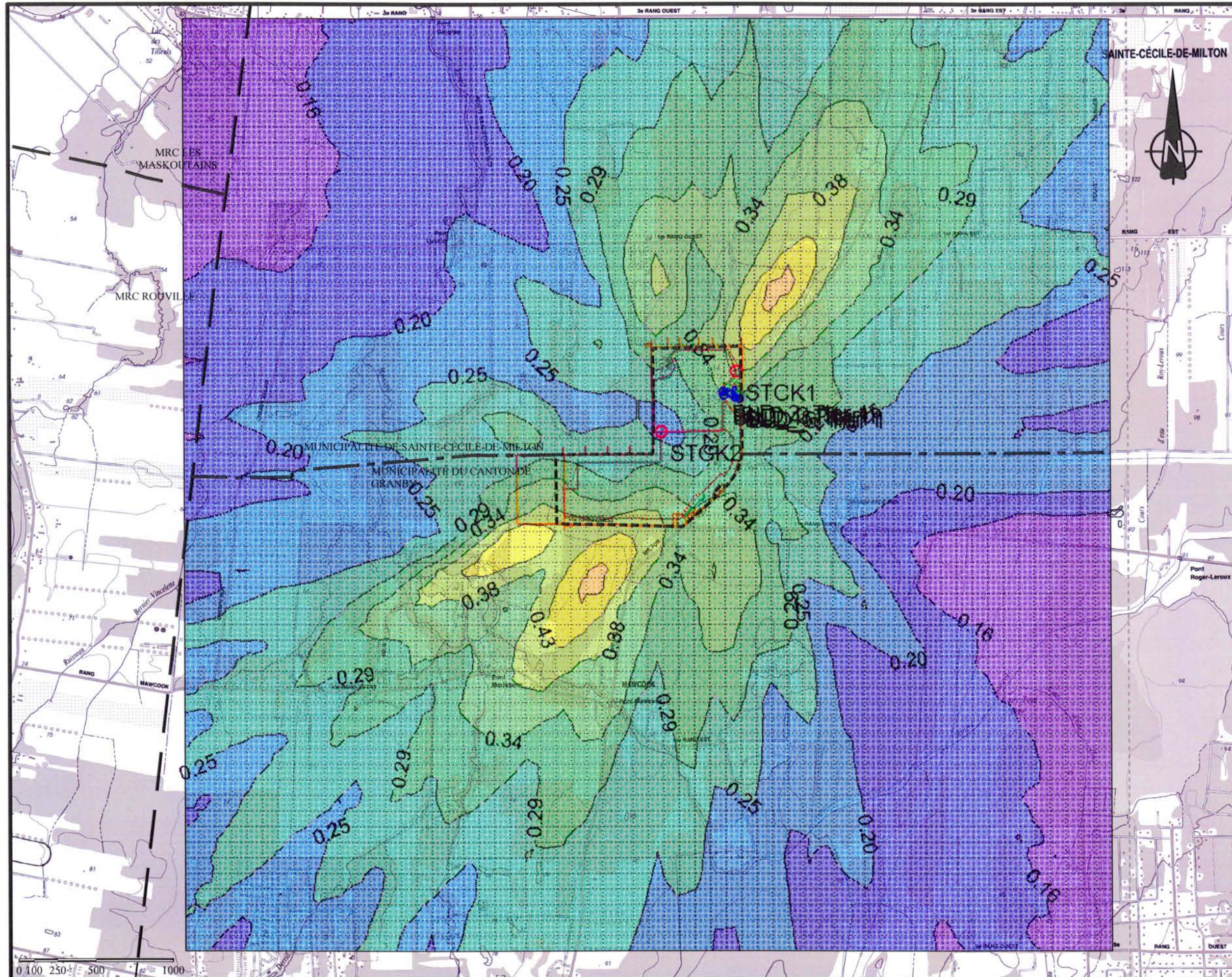
Figure 4.2: Profil de dispersion atmosphérique pour l'année 2042, concentrations maximales horaires des SRT
