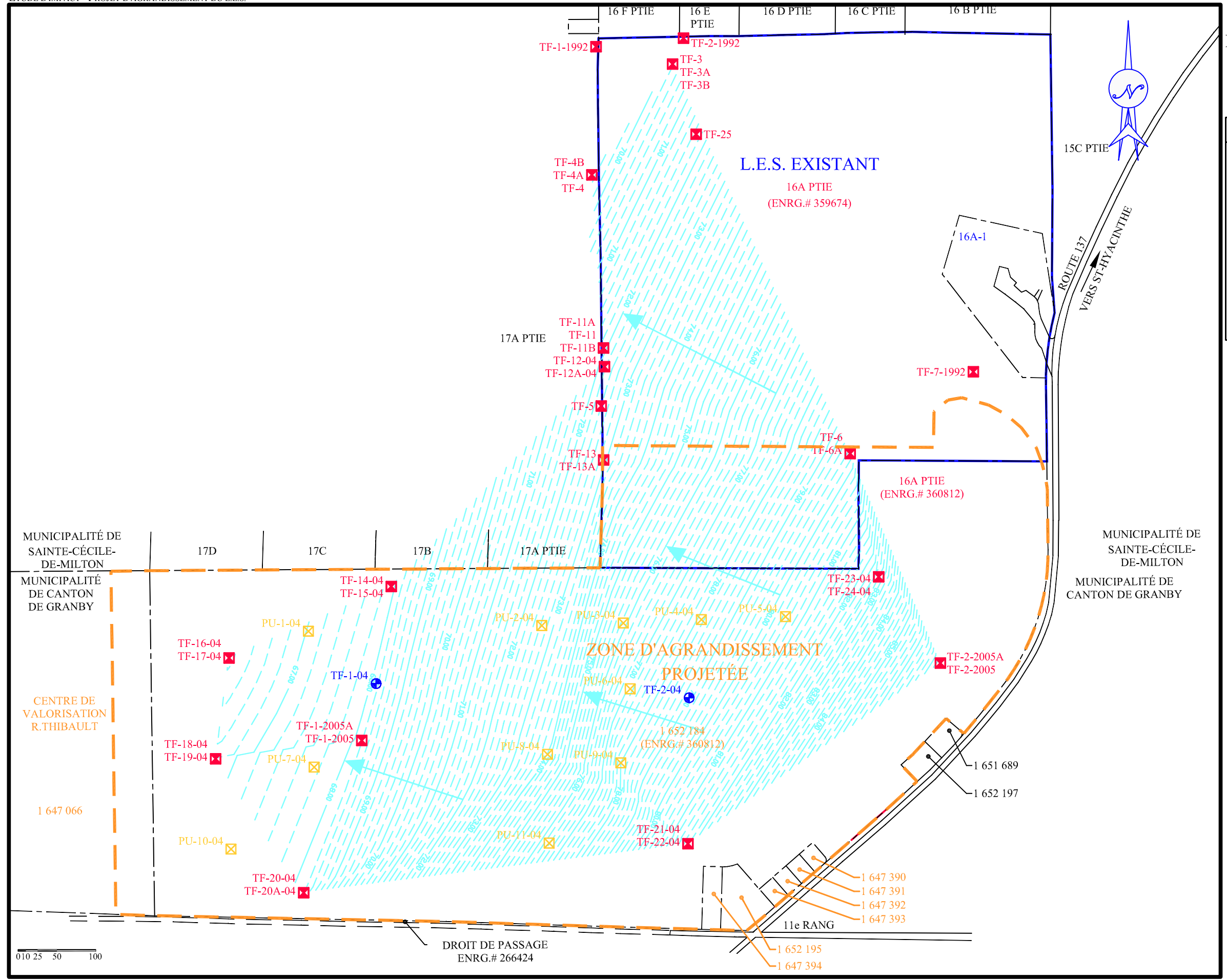
Figure 2.8B: Carte piézométrique - roc fracturé
