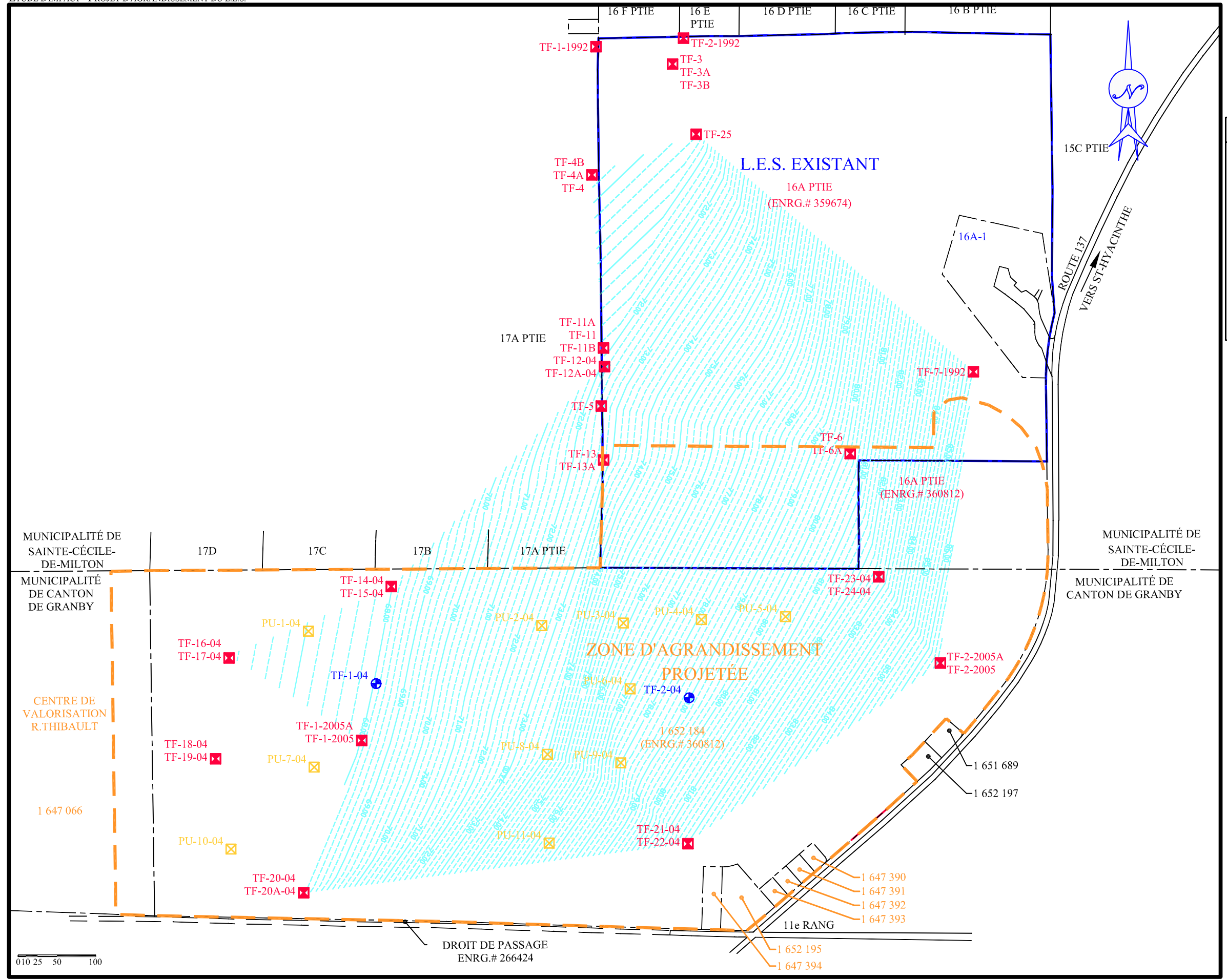
Figure 2.8A: Carte piézométrique - roc sain
