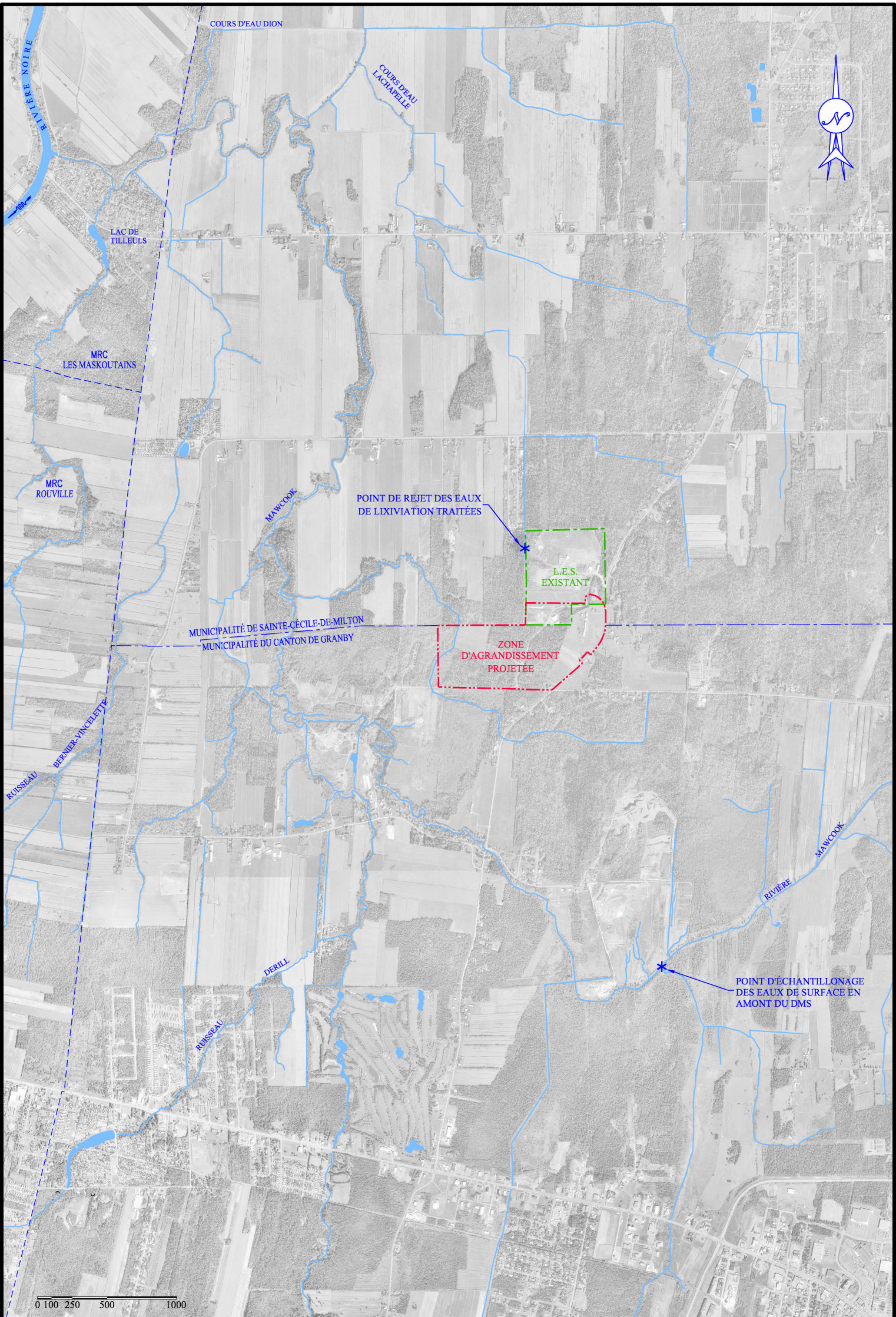
Figure 2.3: Réseau hydrographique du secteur environnant
