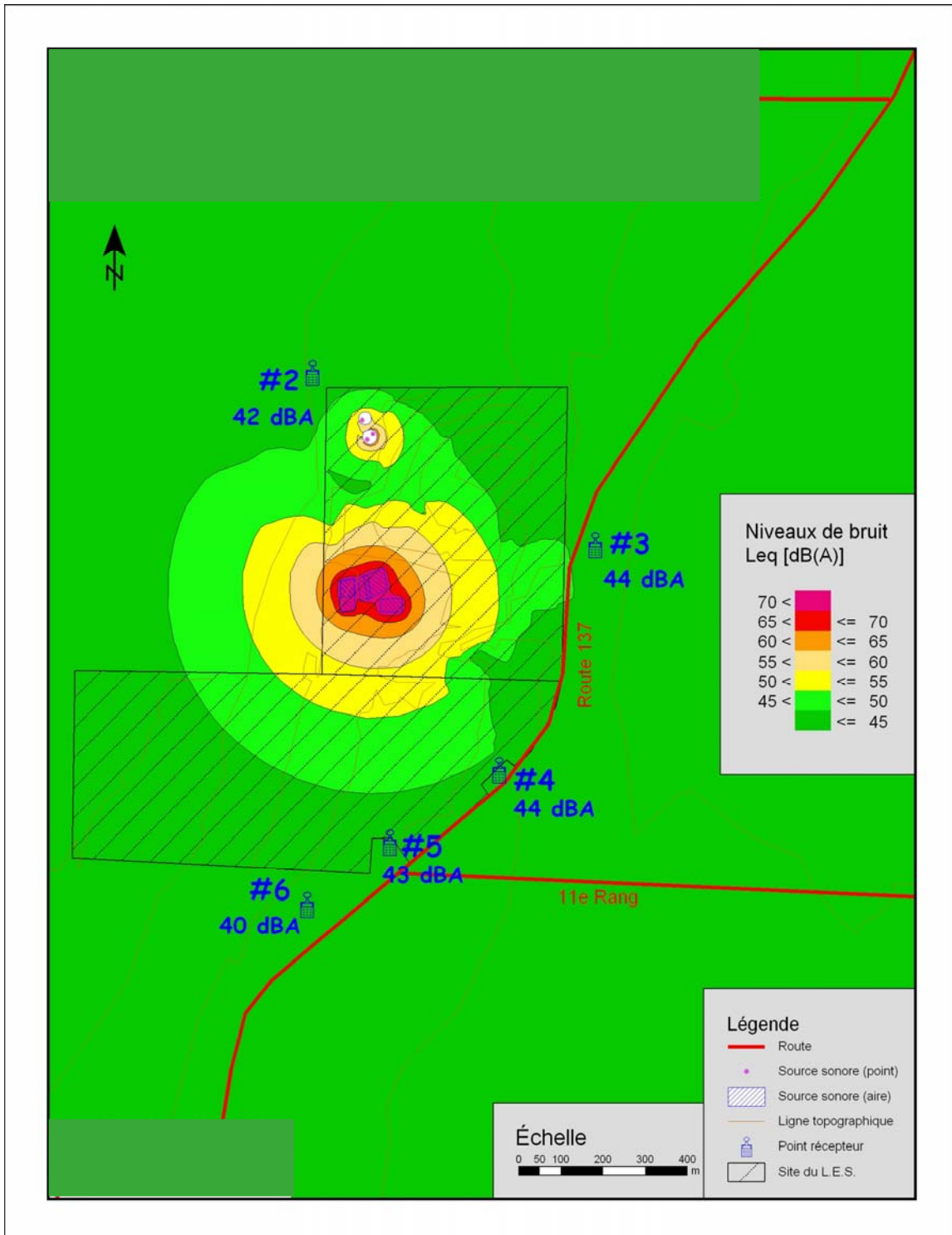
Figure 2.18 : Simulation de propagation du son – Situation actuelle
