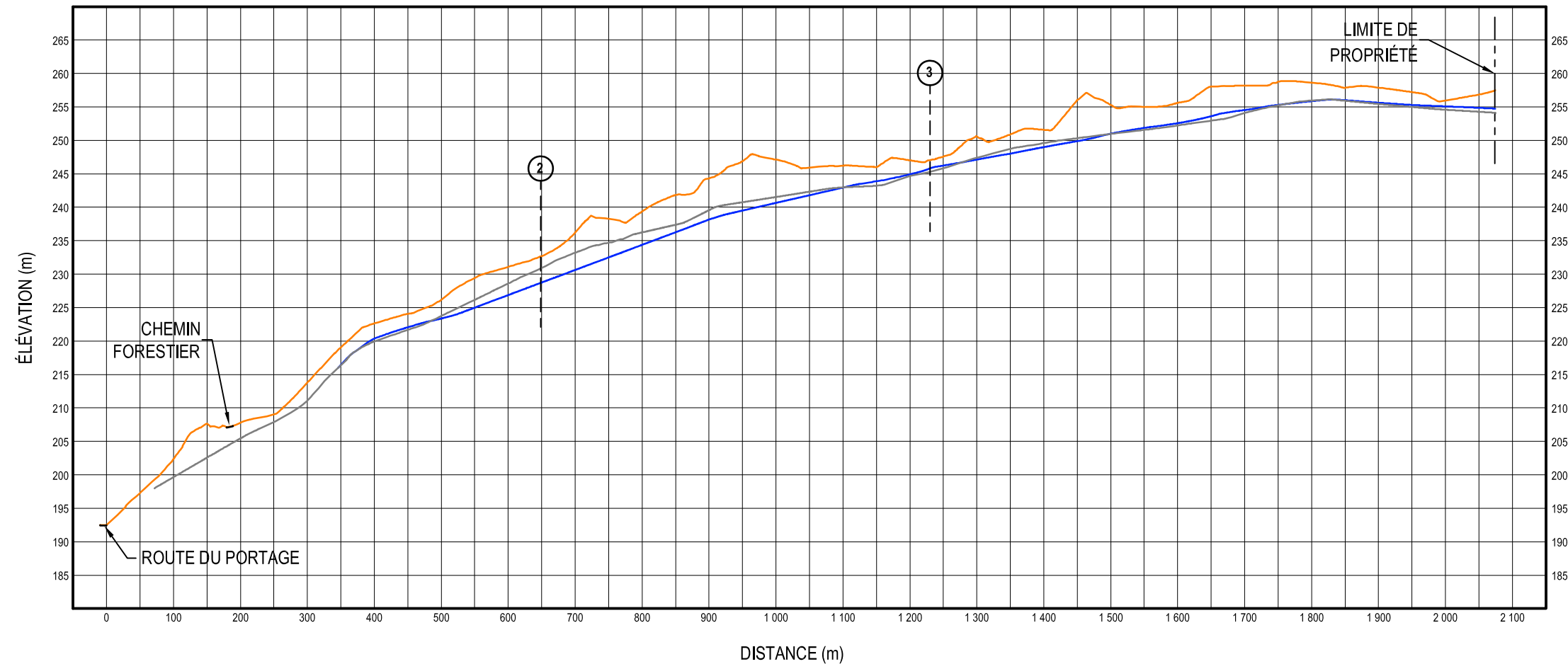
COUPE 1 ÉCHELLE HOR: 1: 8 000 VER: 1: 800
