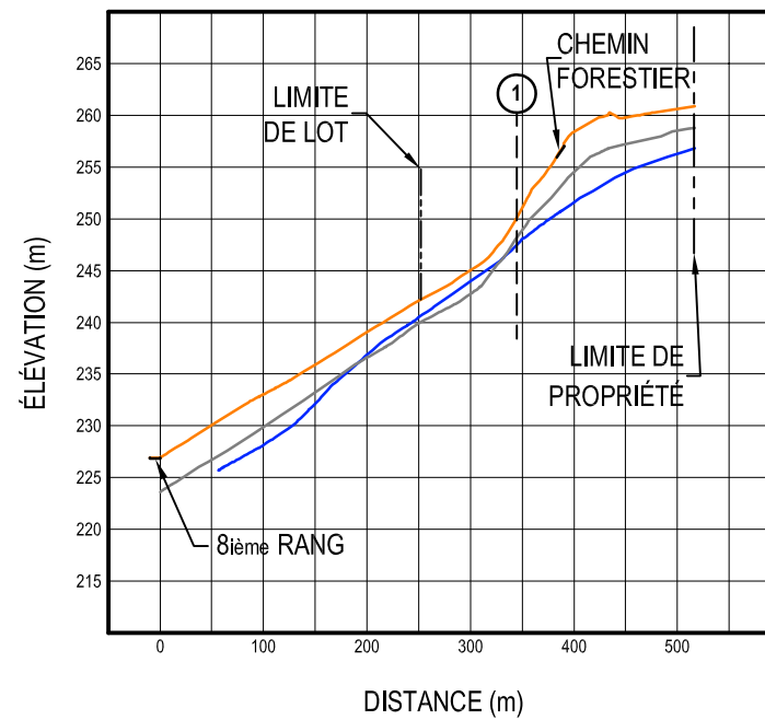
COUPE 3 ÉCHELLE HOR: 1: 8 000 VER: 1: 800
