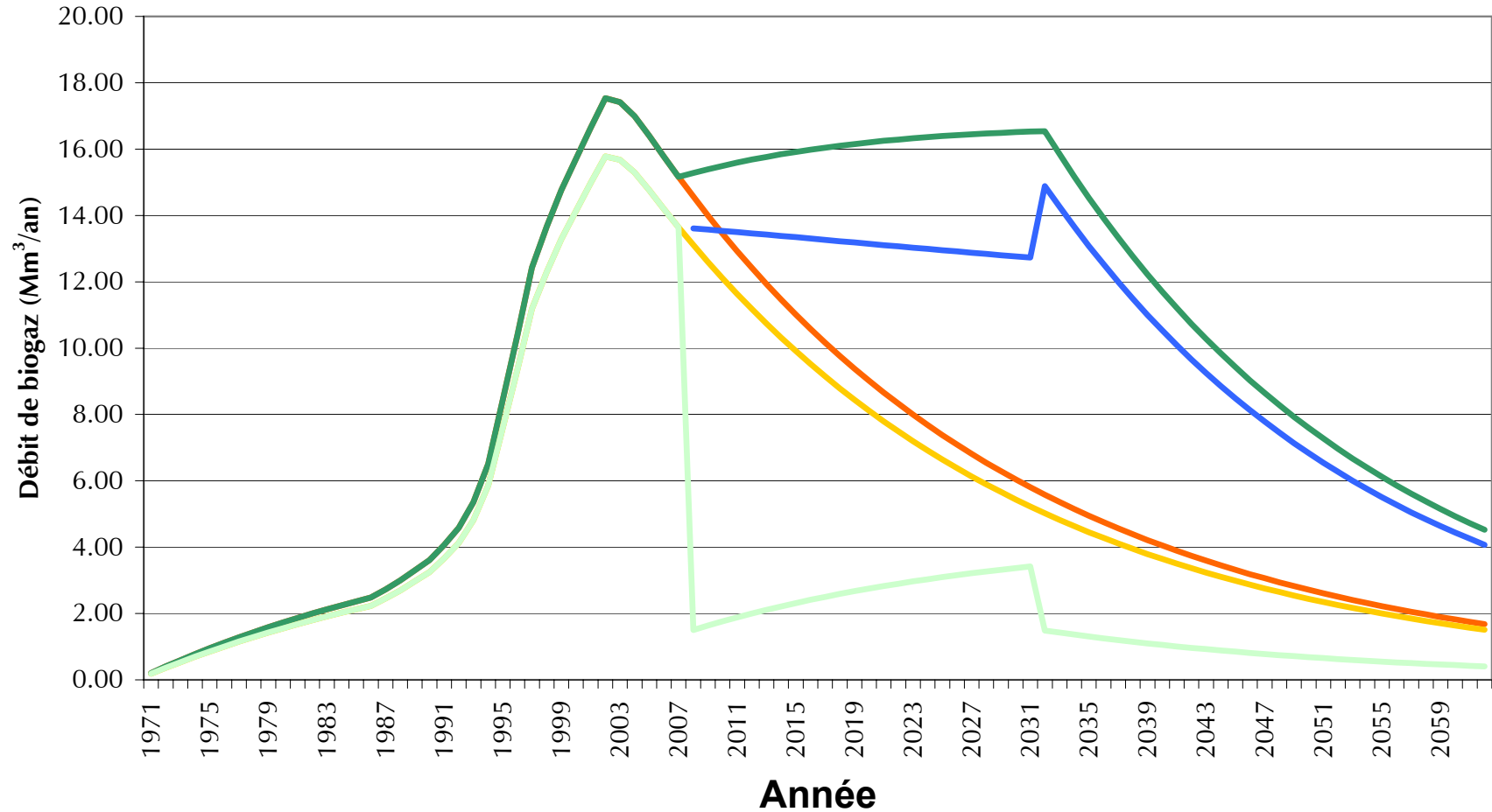
Figure 2.1 Génération et captage du biogaz Situation actuelle et projet proposé
