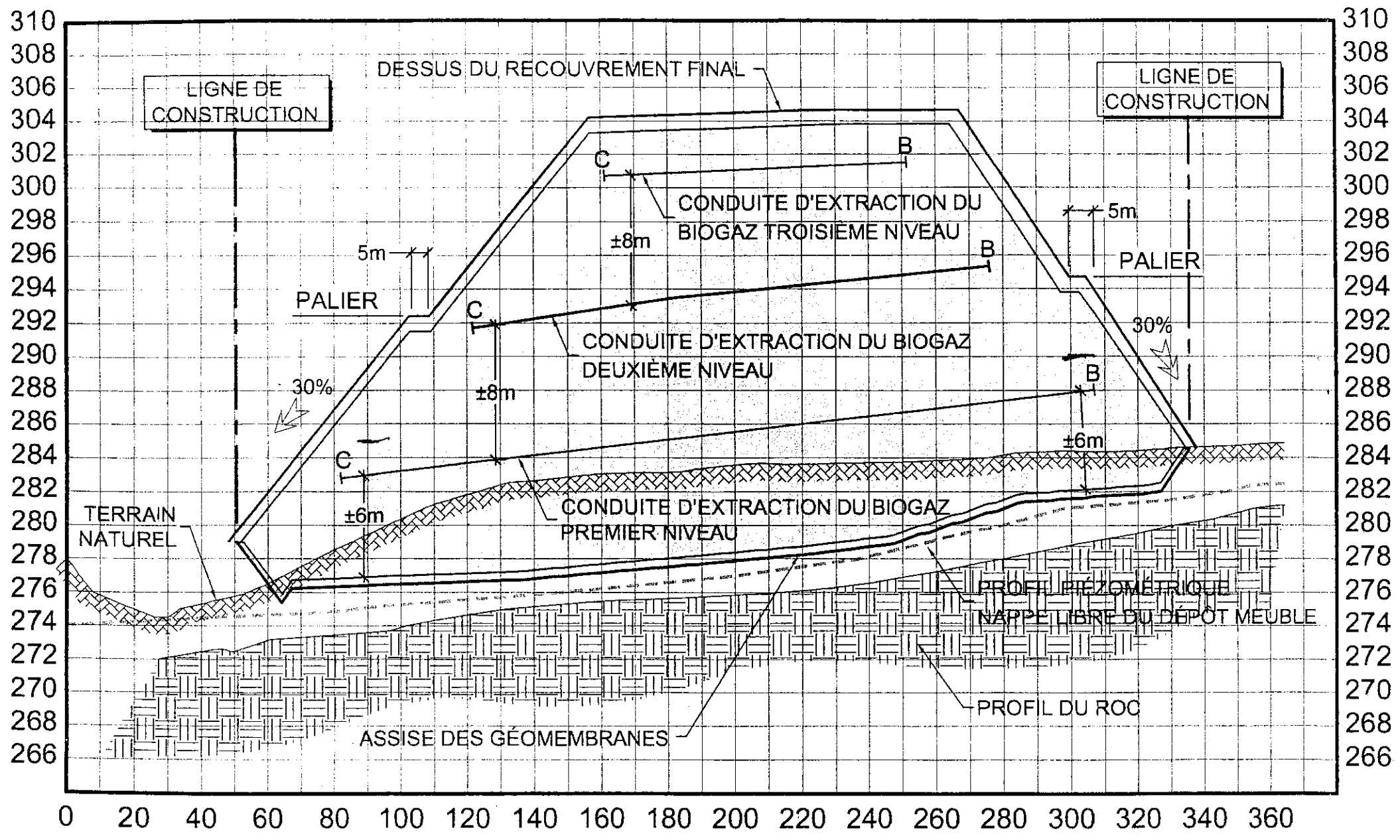
1915039 SECTION NORD SUD (E) ÉCHELLE hor. 1=1500 ver. 1=300
