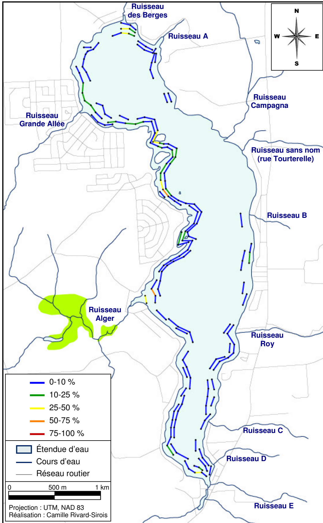
Figure 28 : Recouvrement (%) du myriophylle à épi ( M. spicatum ) dans chaque transect
