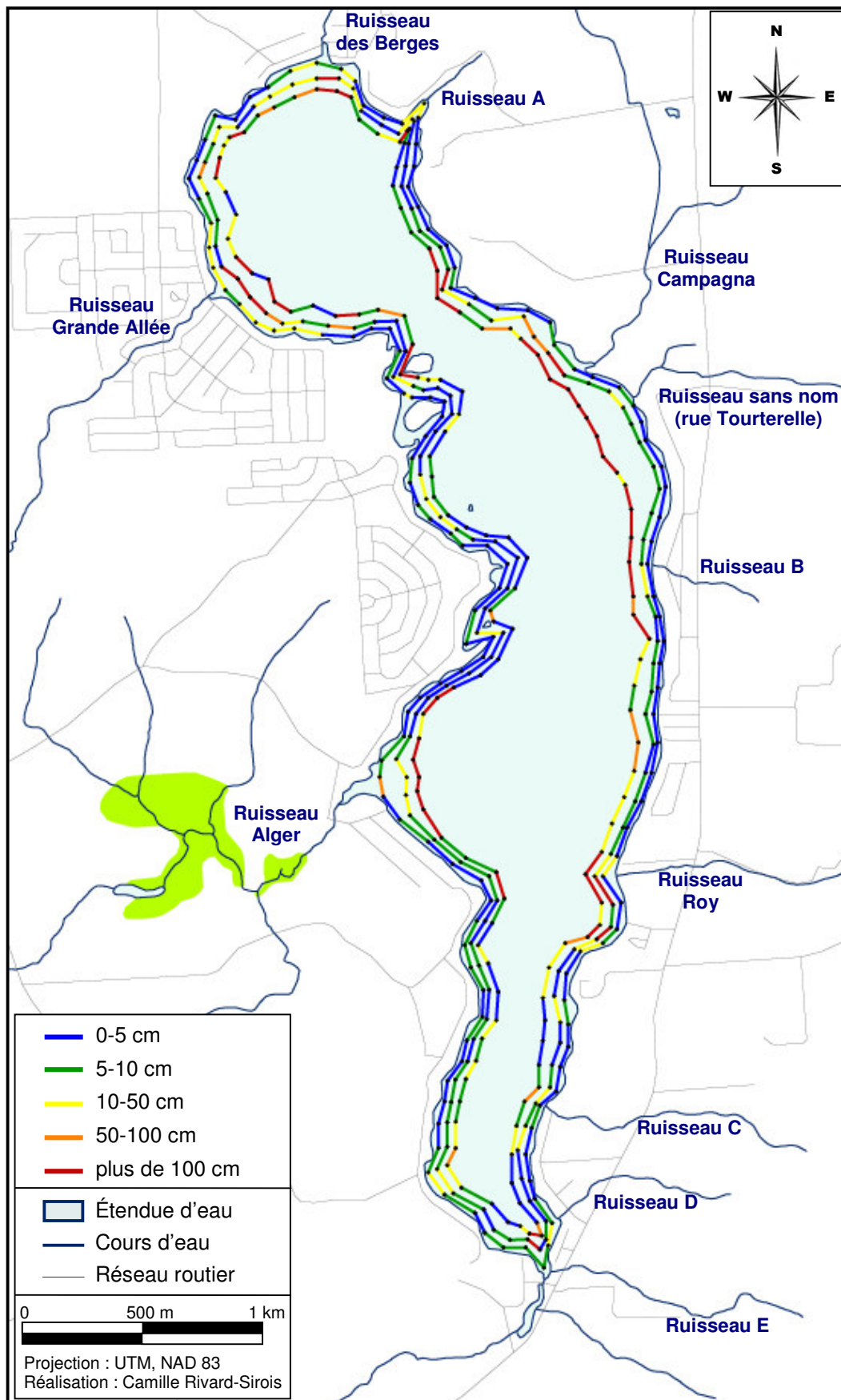
Figure 23 : Épaisseur des sédiments (médiane) dans chaque transect
