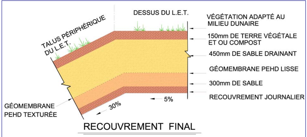
FIGURE 9 – COUPE-TYPE DU RECOUVREMENT FINAL
