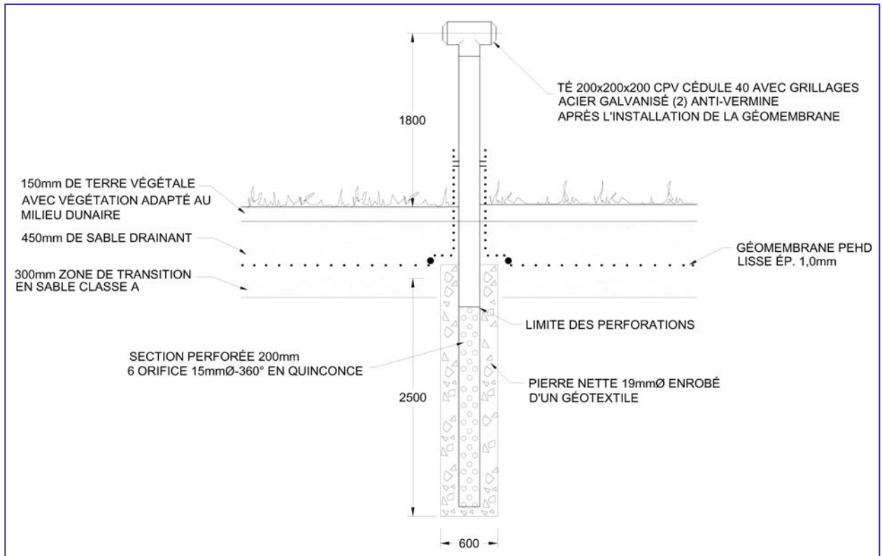
FIGURE 10 – ÉVENT PASSIF TYPE
