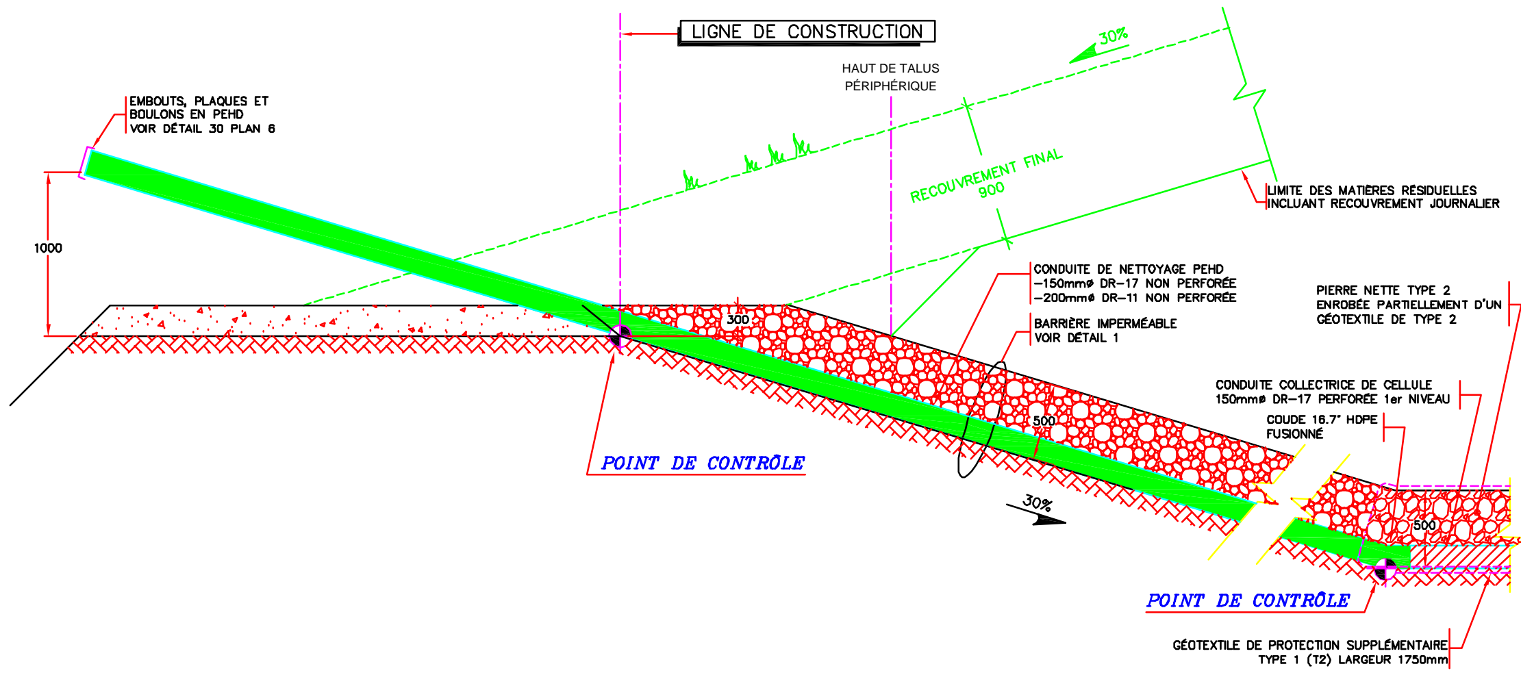
04-1804fig09 DÉTAIL TYPE CONDUITE DE NETTOYAGE Échelle aucune
