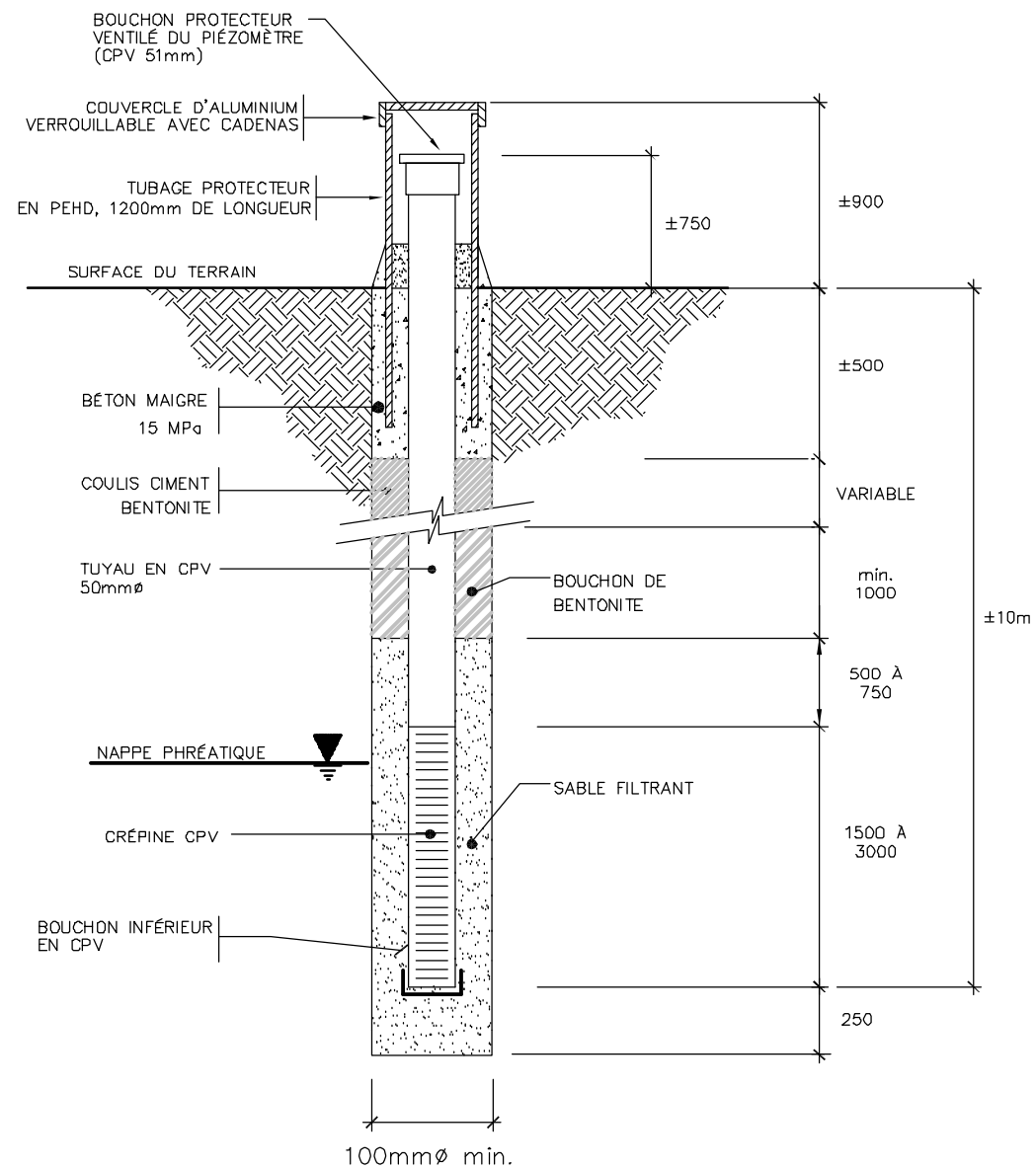
041804fig12 PUITS D'OBSERVATION DES EAUX SOUTERRAINES
