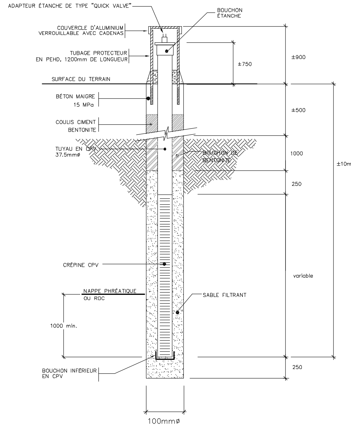
041804fig13 PUITS D'OBSERVATION DES BIOGAZ
