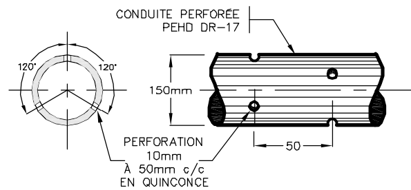
CONDUITE COLLECTRICE 2ième NIVEAU CONDUITE COLLECTRICE DE CELLULE
