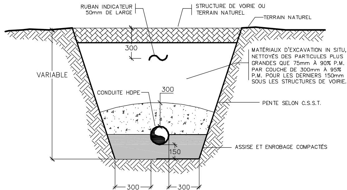
041804fig15 TRANCÉE TYPE UNE CONDUITE HORS CELLULES DE LA ZONE IMPERMÉABILISÉE Echelle aucune
