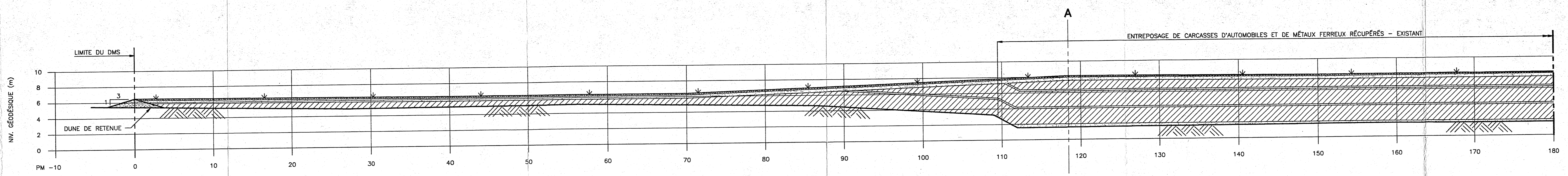
COUPE H-H - PROFIL LONGITUDINAL PM -10 À PM 180 HORZ. 1:200 VERT. 1:200
