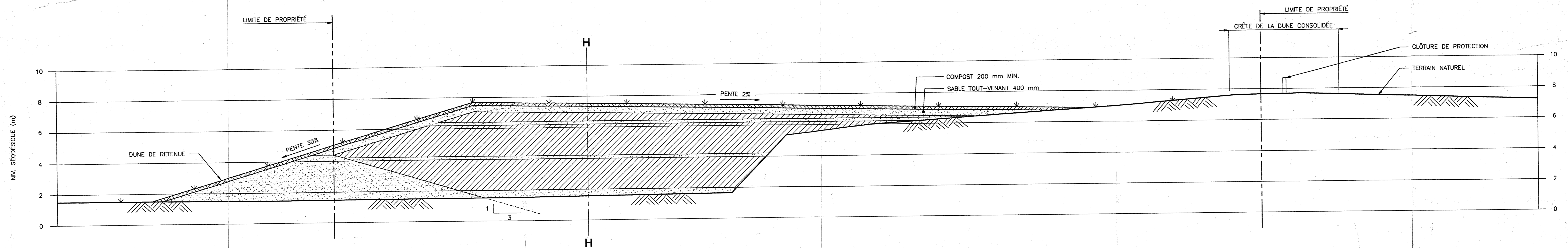
COUPE A-A - COUPE TRANSVERSALE HORZ. 1:100 VERT. 1:100
