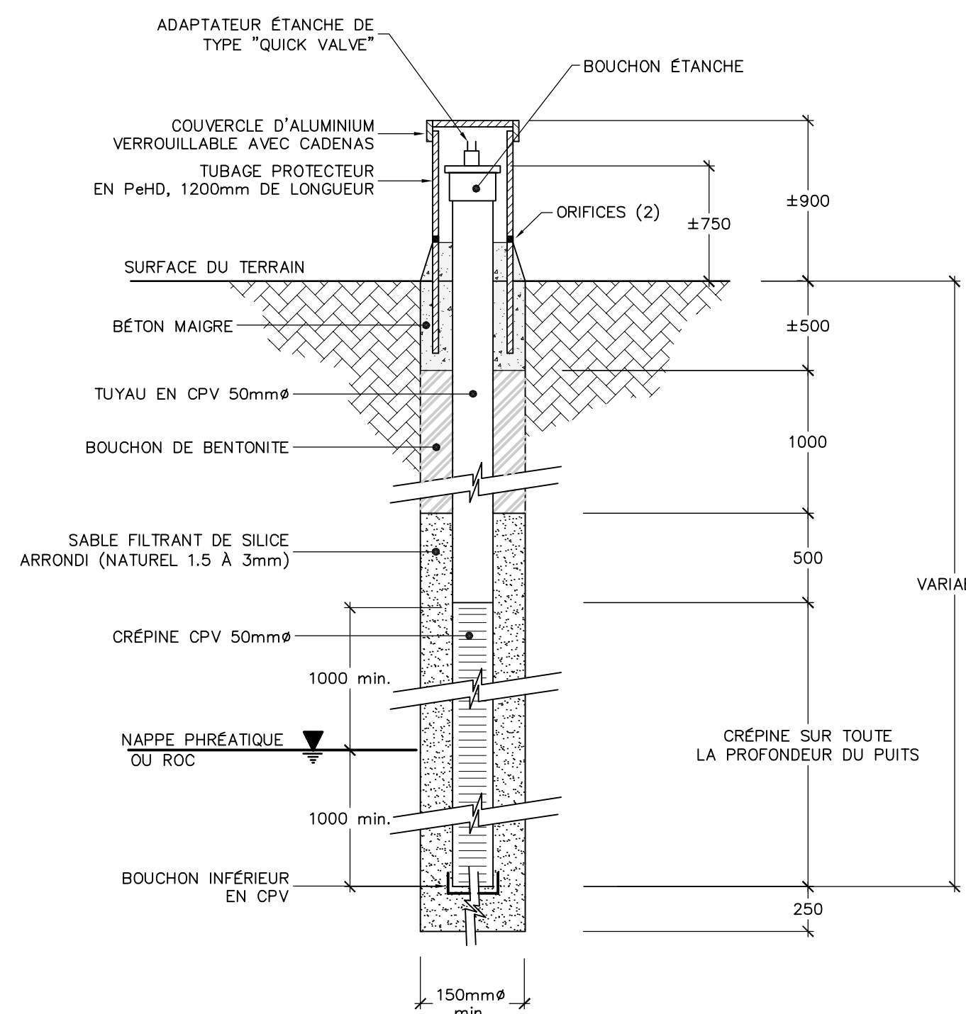
PUITS D'OBSERVATION (SB) DES BIOGAZ TYPIQUE (44) Echelle: aucune
