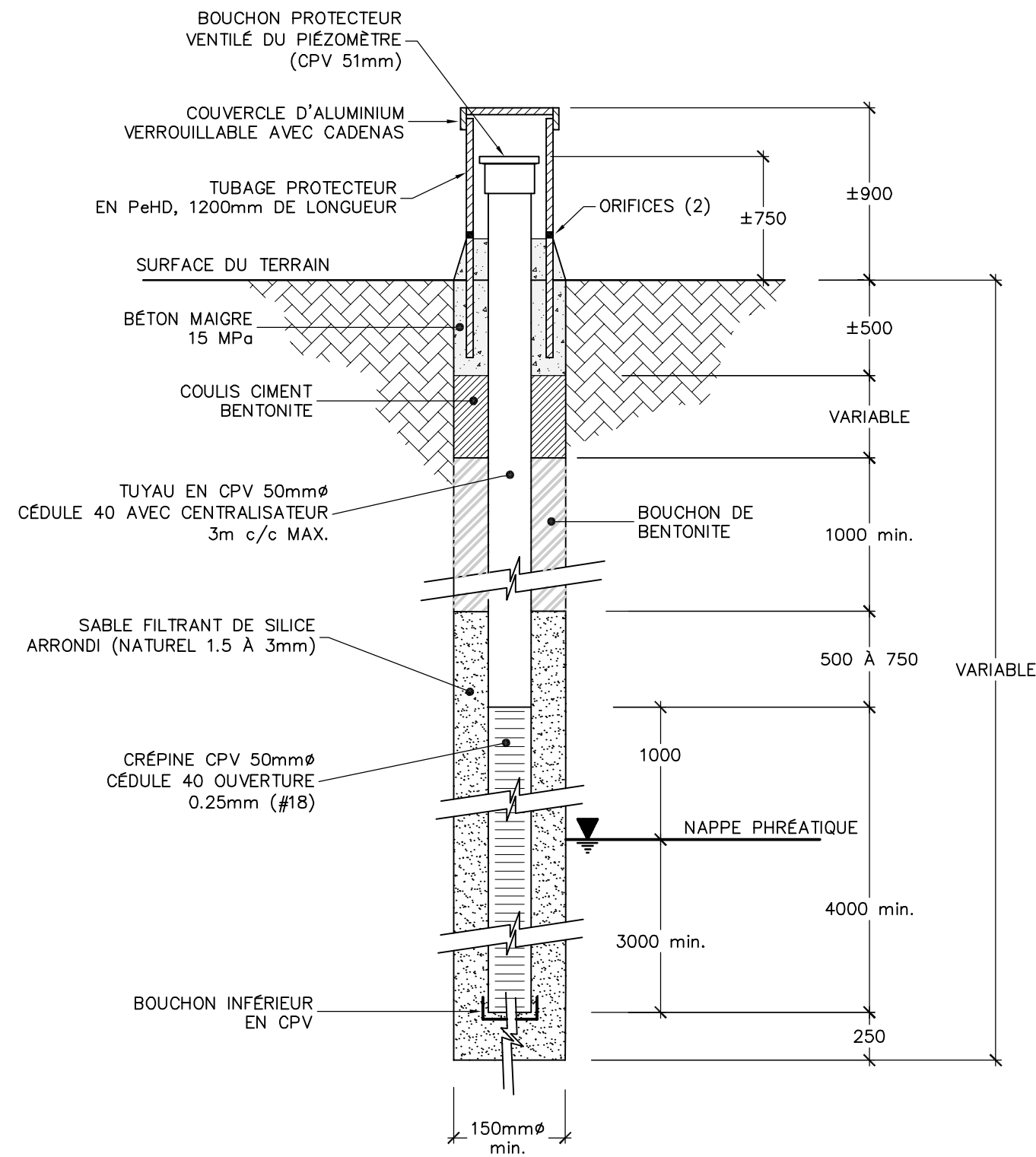
PUITS D'OBSERVATION DES EAUX SOUTERRAINES TYPIQUE (43) Echelle: aucune
