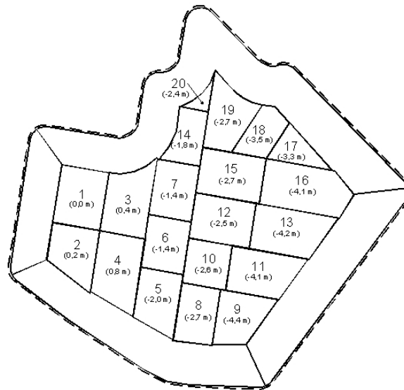
Figure 4 Plan de la future cellule d'enfouissement
