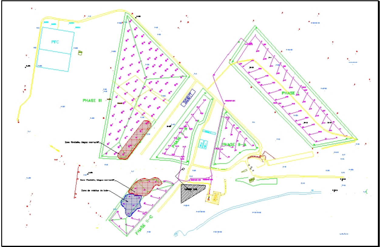
Figure 3 Plan du site
