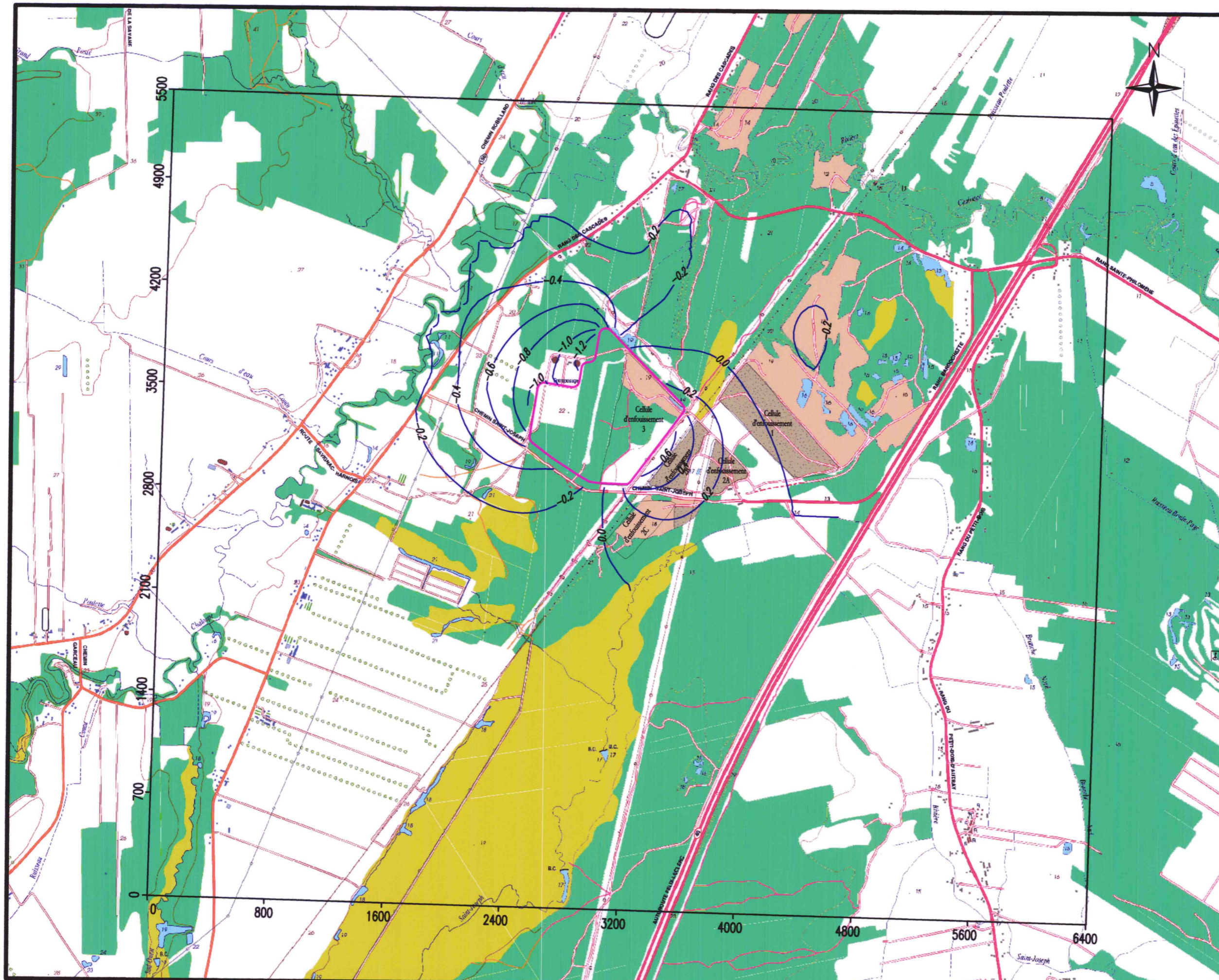
Figure 6.4 : RABATTEMENT SIMULÉ DE LA NAPPE LIBRE AVEC LA NOUVELLE CELLULE APRÈS 35 ANS
