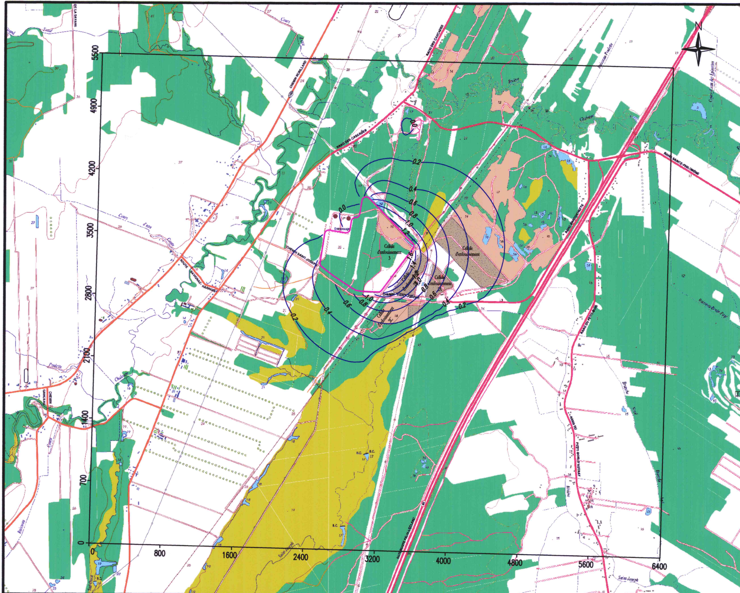
Figure 6.2 : RABATTEMENT SIMULÉ DE LA NAPPE LIBRE AVEC LA NOUVELLE CELLULE APRÈS 5 ANS
