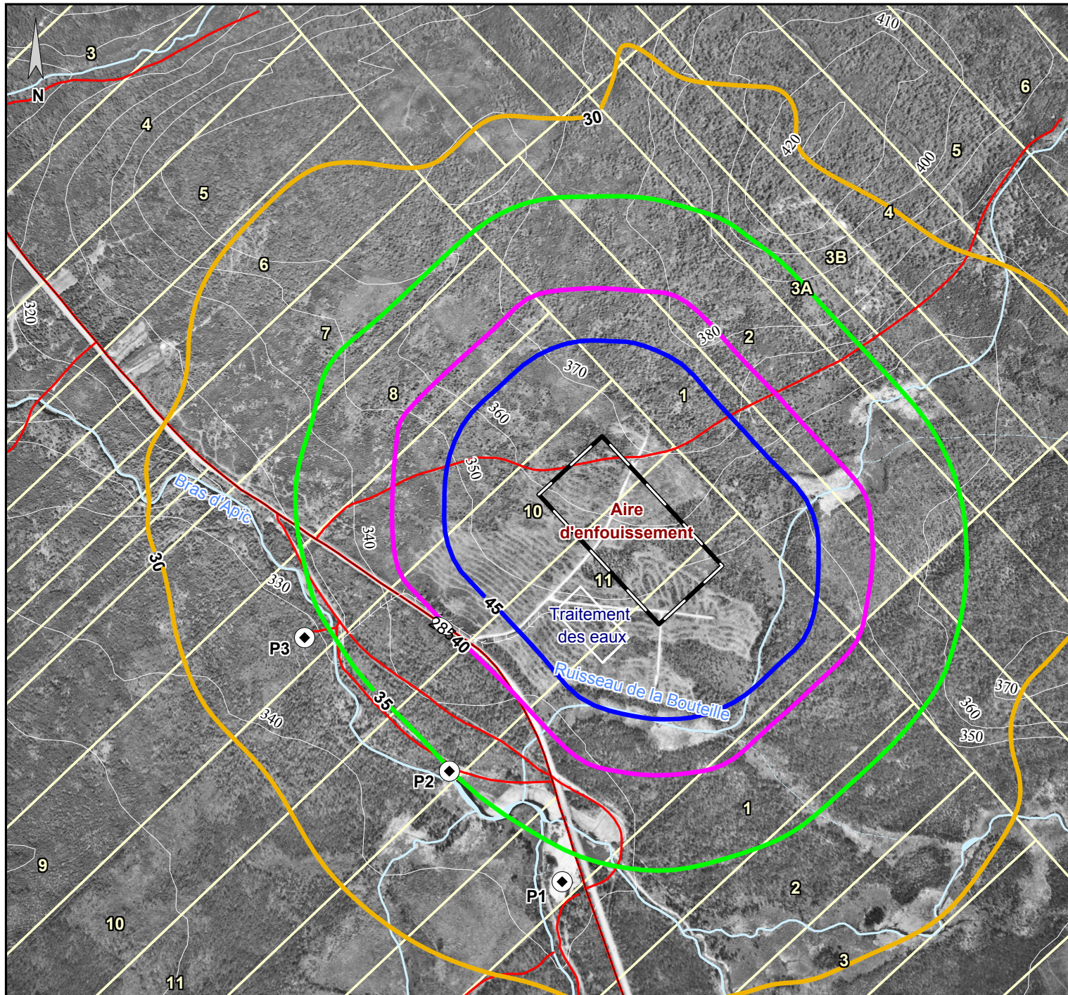
Figure 5.2 Isophones Leq, 1h de l'exploitation du LET
