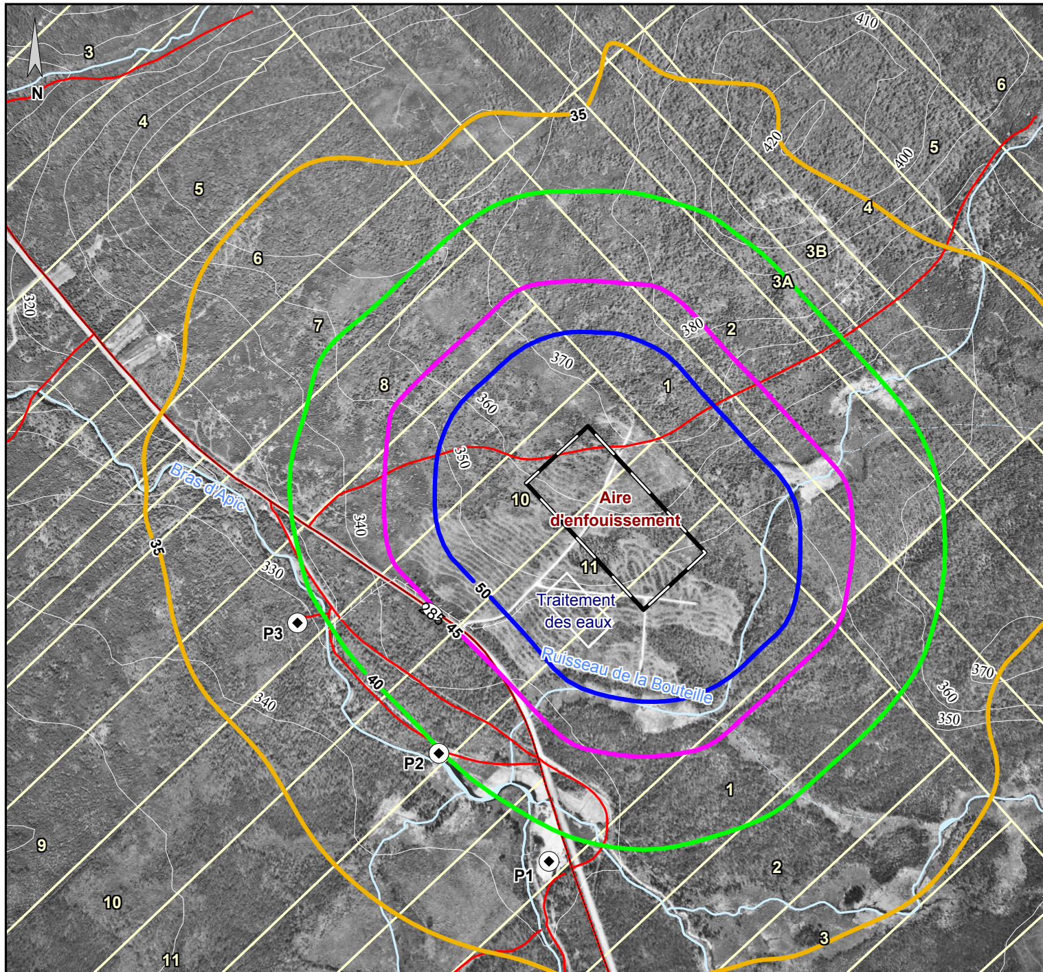
Figure 5.1 Isophones Leq, 1h de la construction de la phase I
