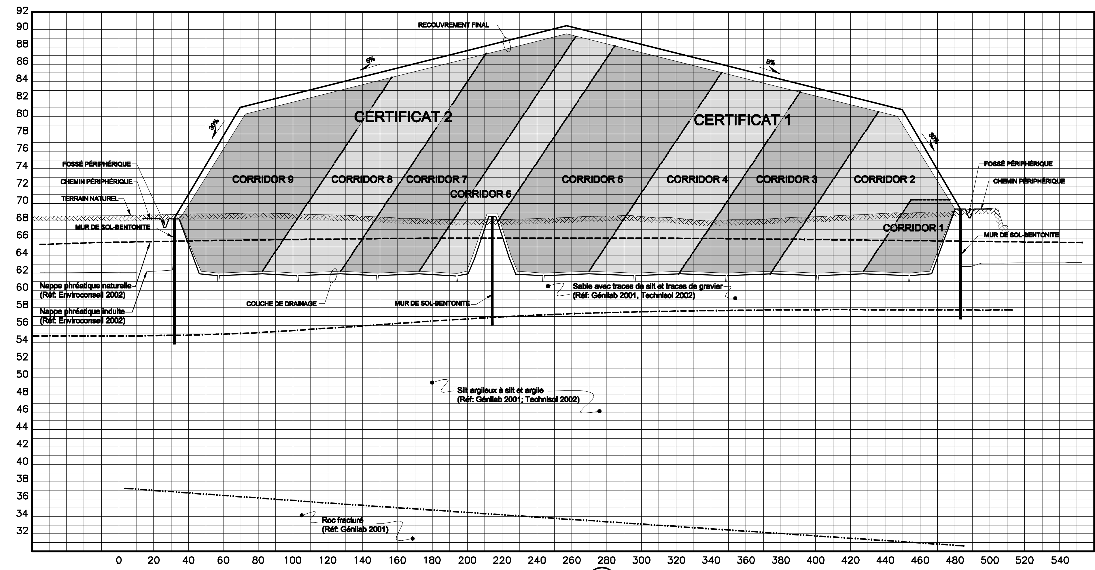
COUPE TRANSVERSALE B 6/4
