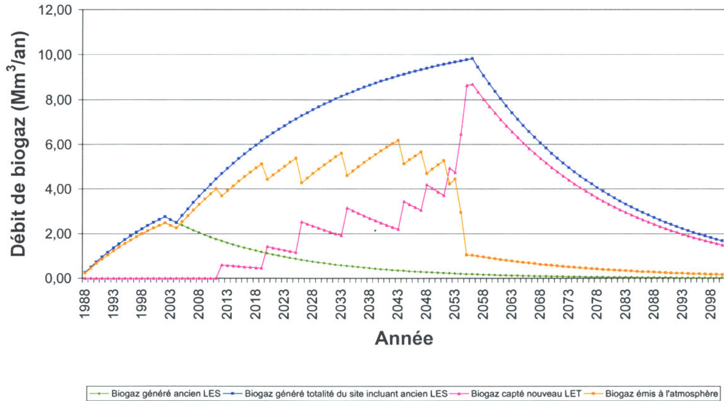
Figure 2-2 : Modélisation de la génération et du captage du biogaz - LES et LET de Matane
