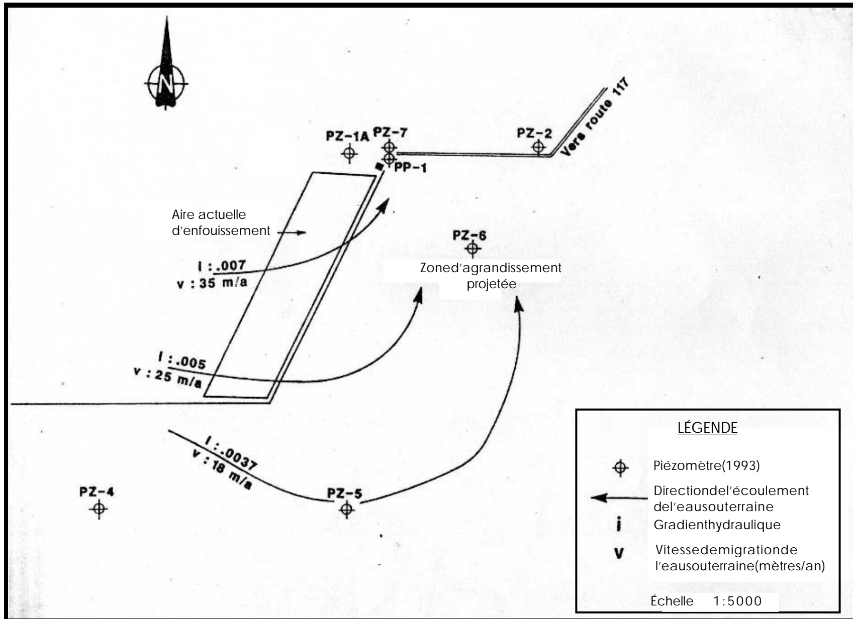
Figure 4.2 Localisation des piézomètres sur le site d'enfouissement sanitaire de Marchand.
