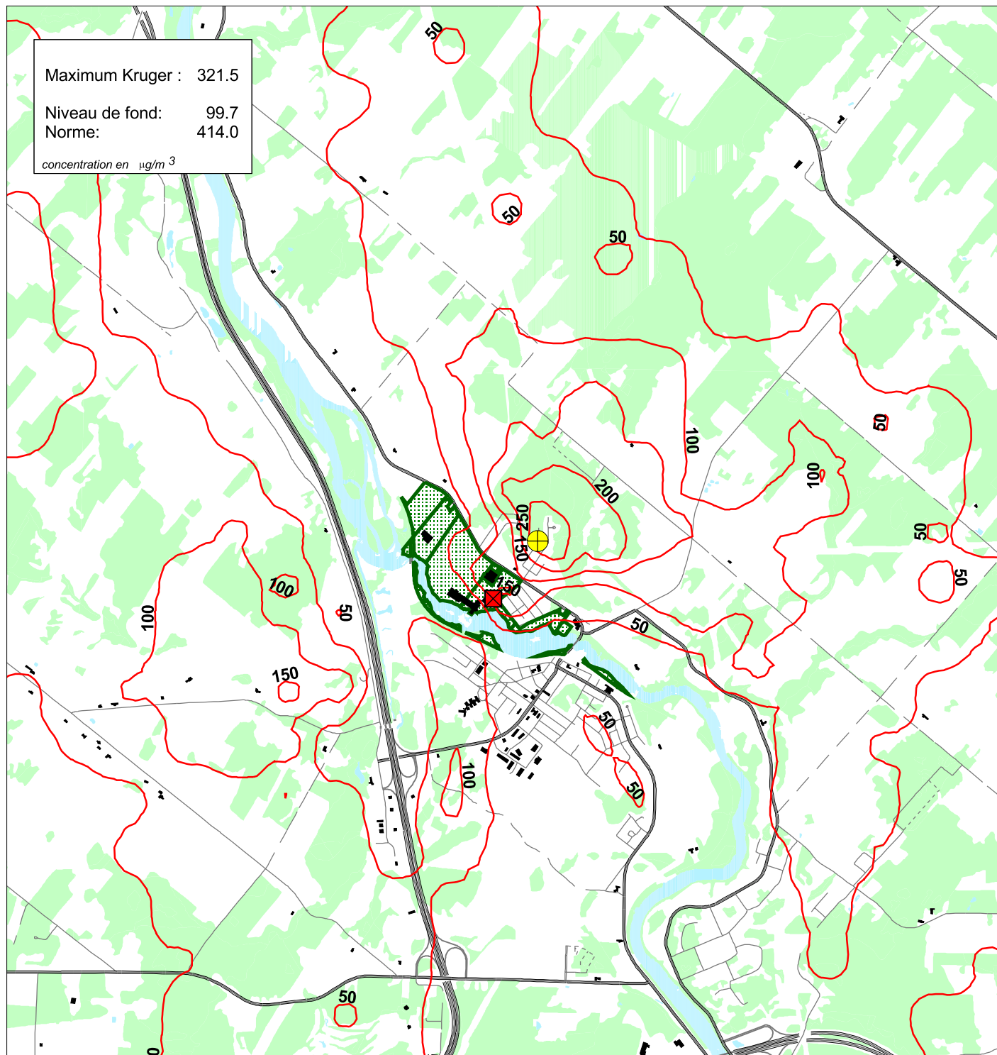
Figure 9 : Zone d'influence du NO2 - pire cas sur 1 heure Situation actuelle
