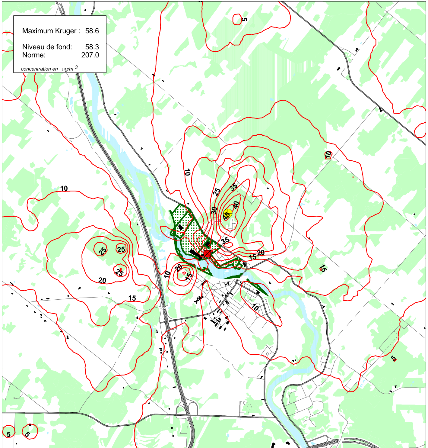
Figure 6 : Zone d'influence du NO2 - pire cas sur 24 heures Situation actuelle
