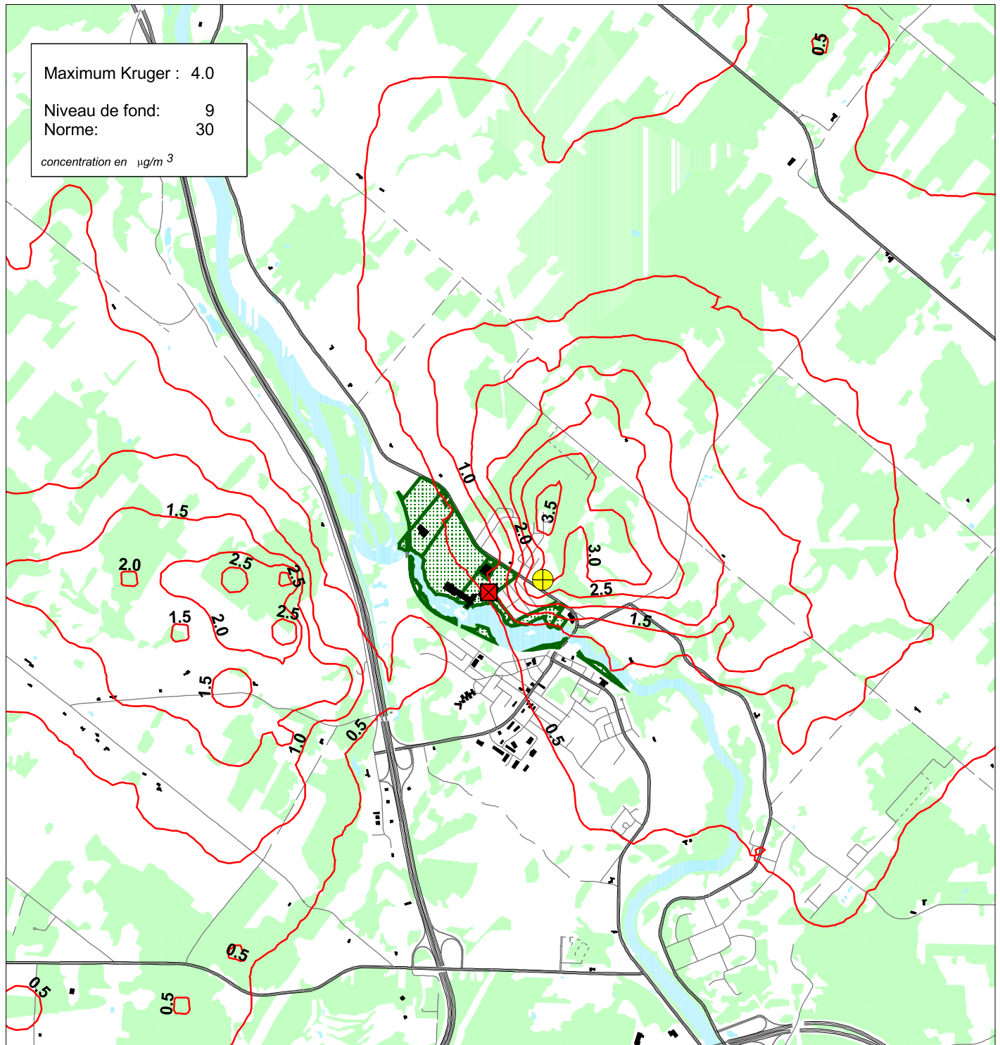
Figure 35 : Zone d'influence des PM 2.5 - pire cas sur 24 heures Situation projetée - scénario 2
