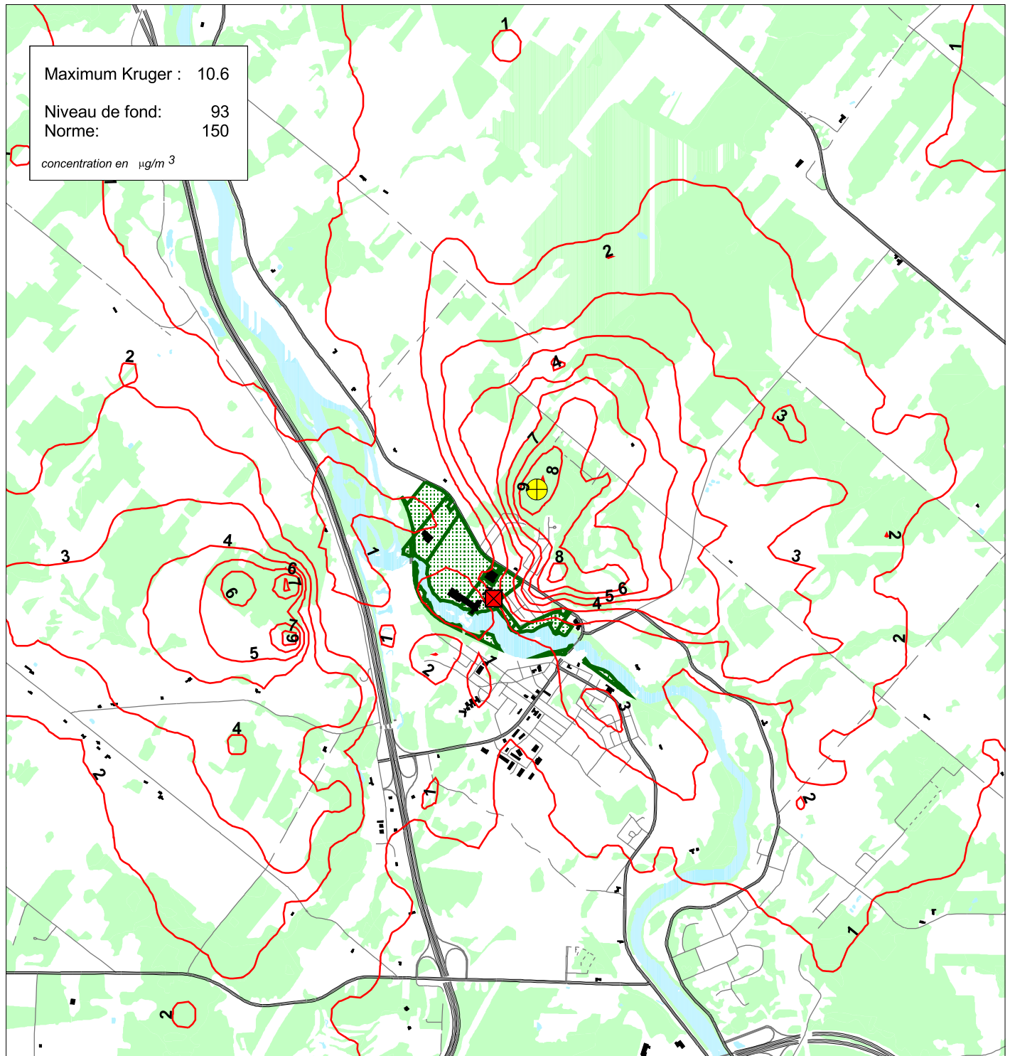
Figure 32 : Zone d'influence des PM - pire cas sur 24 heures Situation projetée - scénario 2
