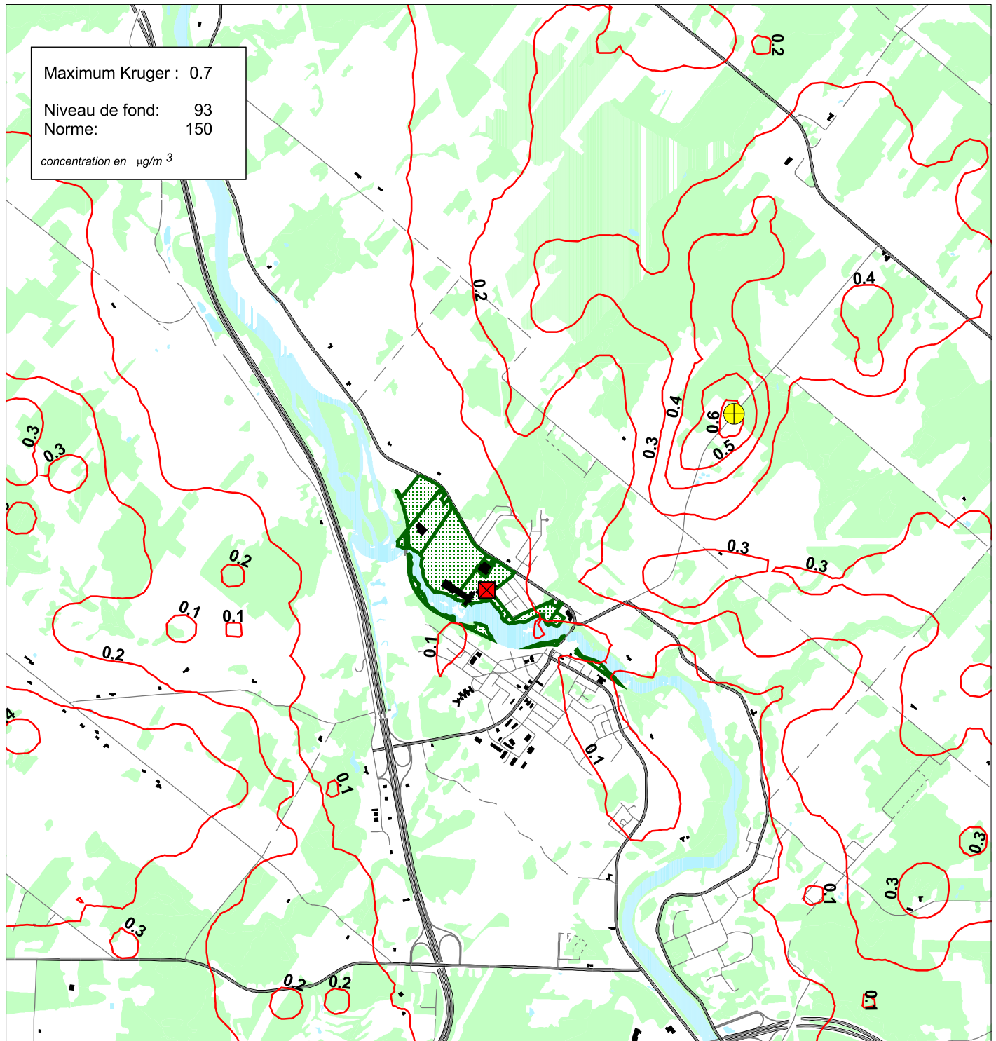
Figure 31 : Zone d'influence des PM - pire cas sur 24 heures Situation projetée - scénario 1
