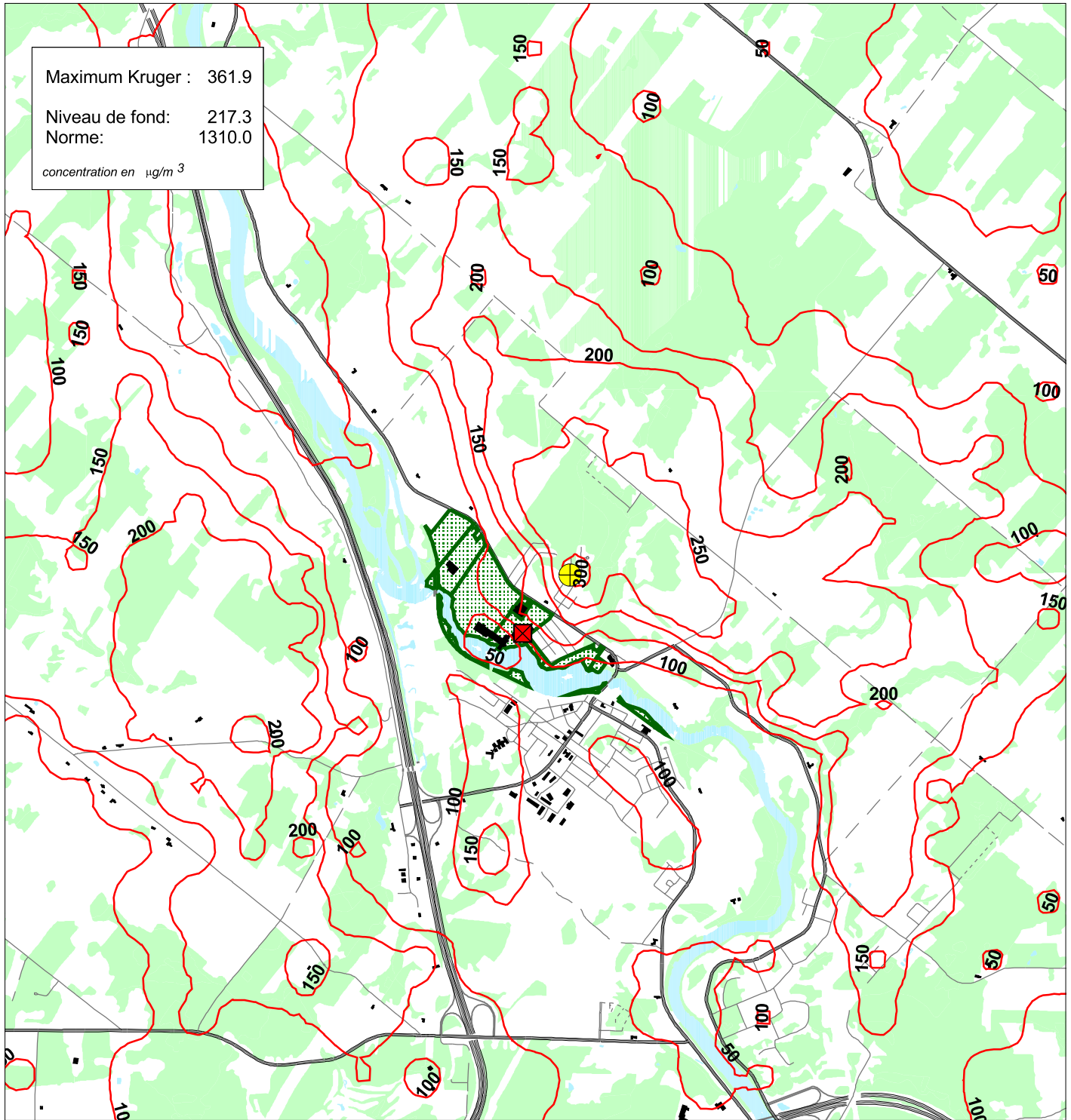
Figure 26 : Zone d'influence du SO 2 - pire cas sur 1 heure Situation projetée - scénario 2
