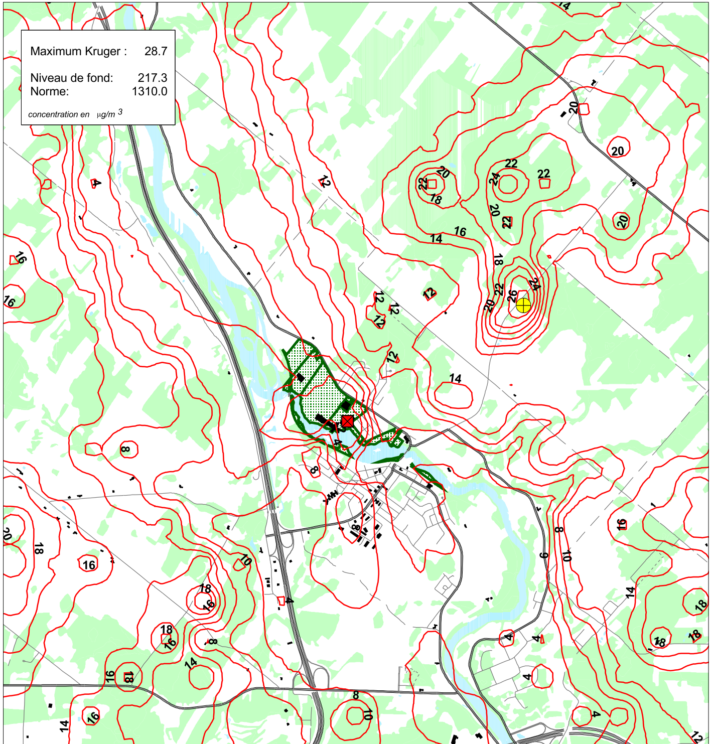
Figure 25 : Zone d'influence du SO 2 - pire cas sur 1 heure Situation projetée - scénario 1
