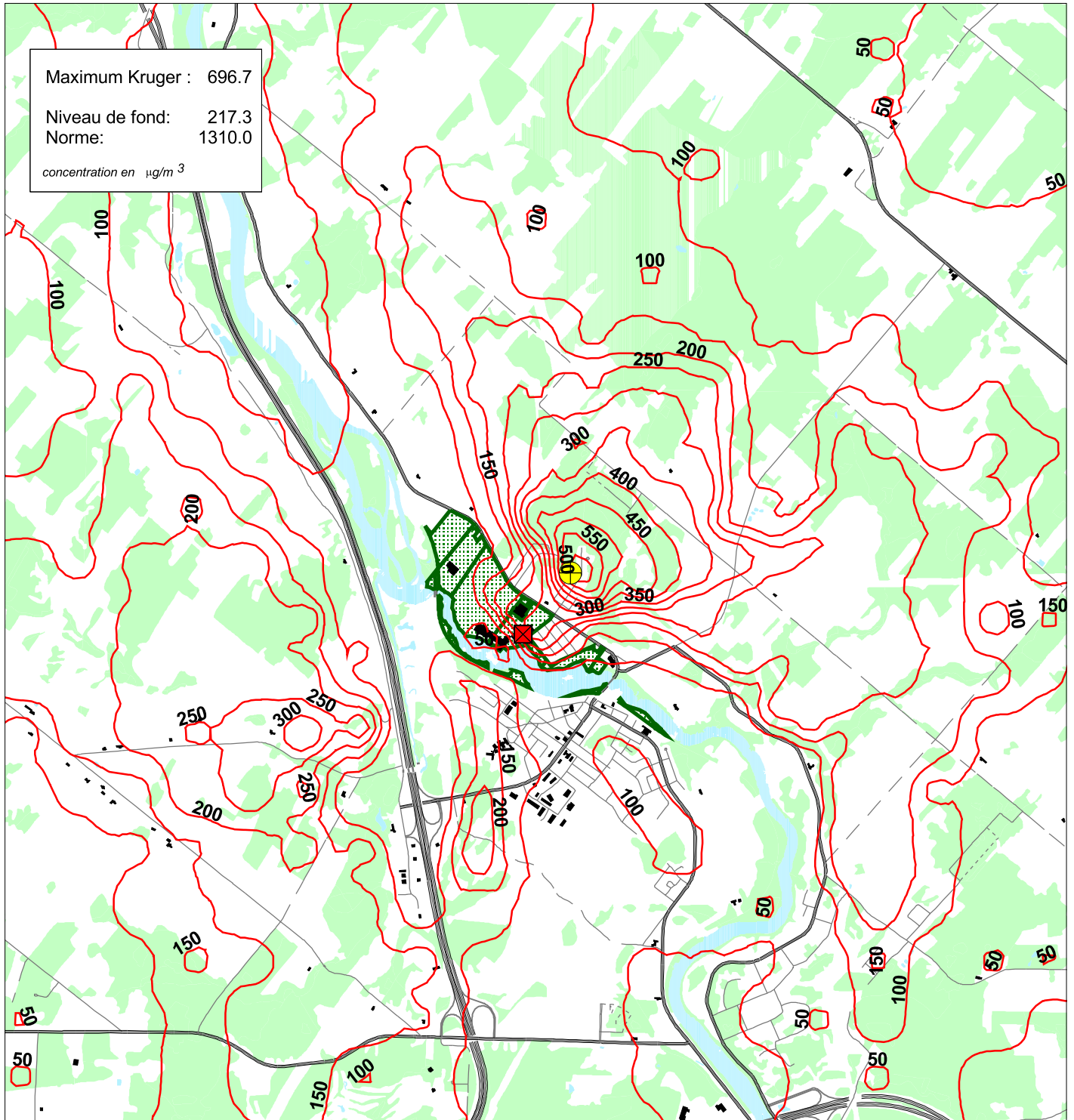
Figure 24 : Zone d'influence du SO 2 - pire cas sur 1 heure Situation actuelle
