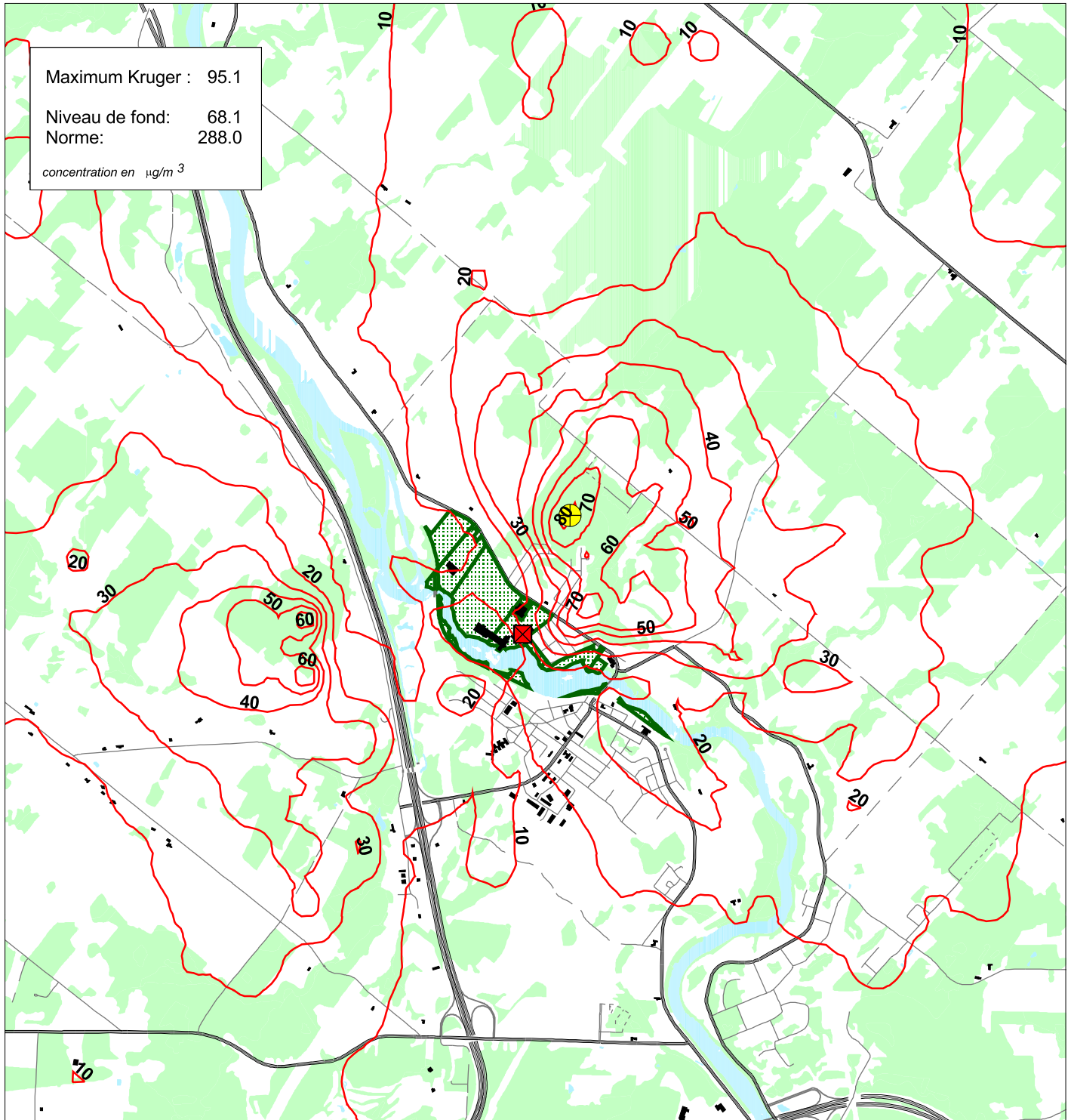
Figure 23 : Zone d'influence du SO 2 - pire cas sur 24 heures Situation projetée - scénario 2
