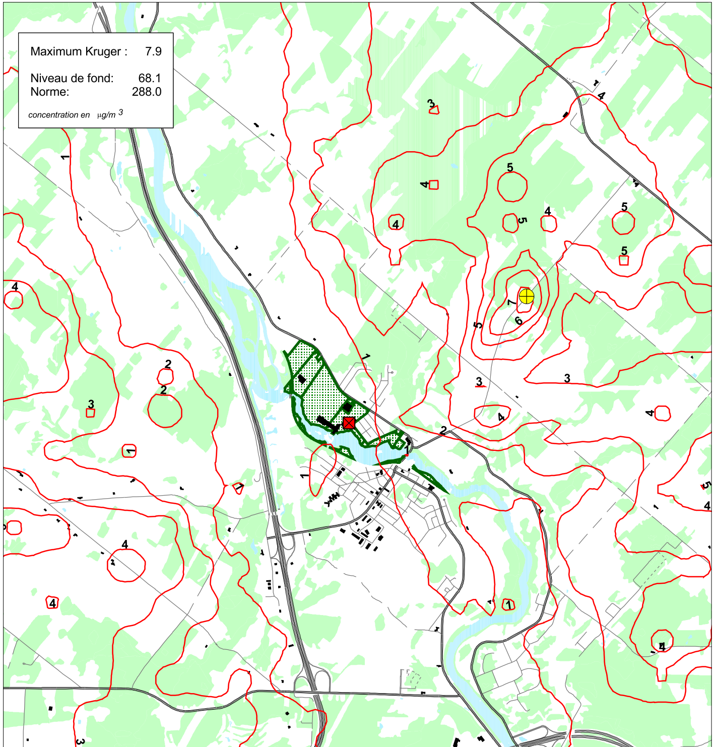
Figure 22 : Zone d'influence du SO 2 - pire cas sur 24 heures Situation projetée - scénario 1
