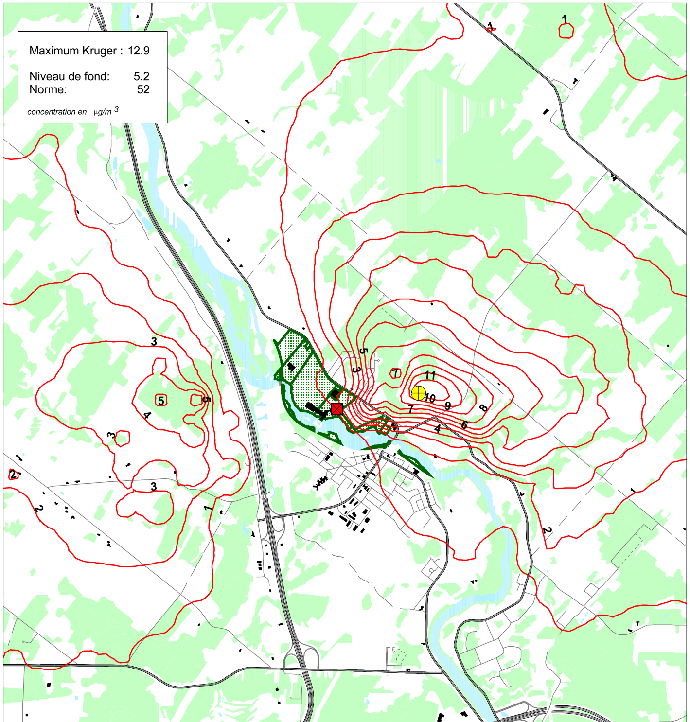
Figure 20 : Zone d'influence du SO 2 - pire cas sur 1 an Situation projetée - scénario 2
