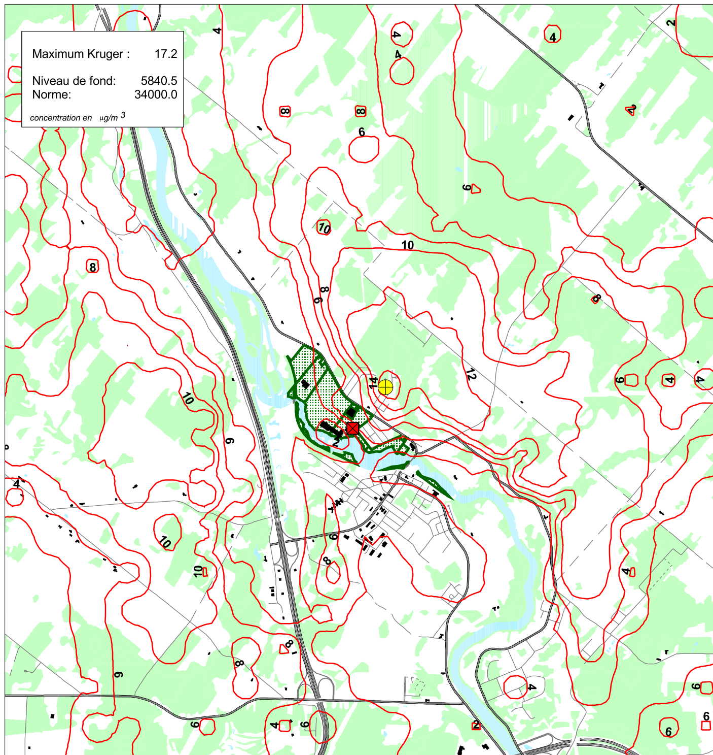
Figure 17 : Zone d'influence du CO - pire cas sur 1 heure Situation projetée - scénario 2
