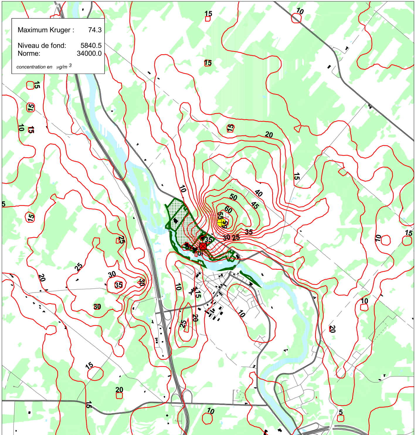
Figure 15 : Zone d'influence du CO - pire cas sur 1 heure Situation actuelle
