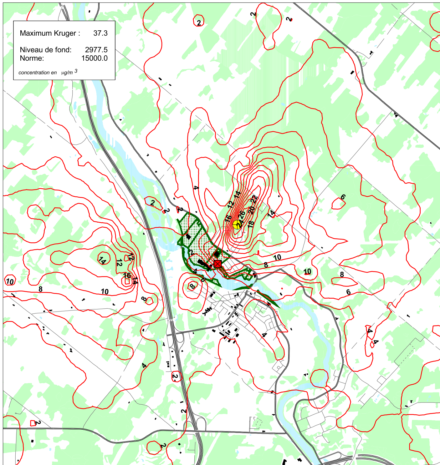
Figure 12 : Zone d'influence du CO - pire cas sur 8 heure Situation actuelle
