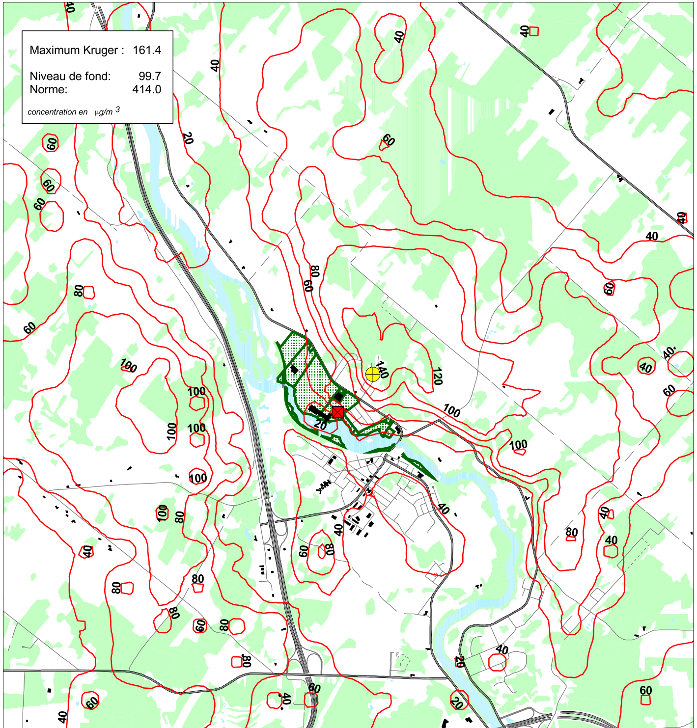
Figure 11 : Zone d'influence du NO2 - pire cas sur 1 heure Situation projetée - scénario 2
