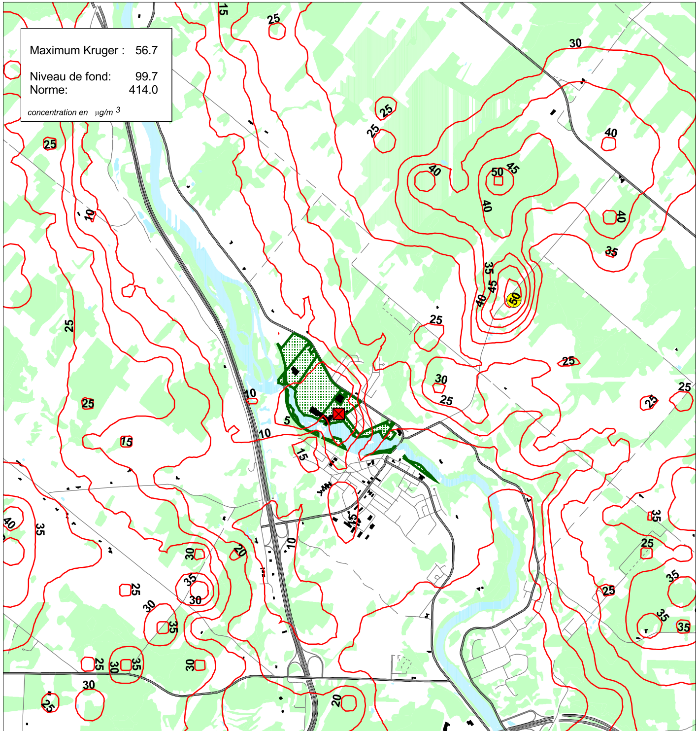
Figure 10 : Zone d'influence du NO2 - pire cas sur 1 heure Situation projetée - scénario 1
