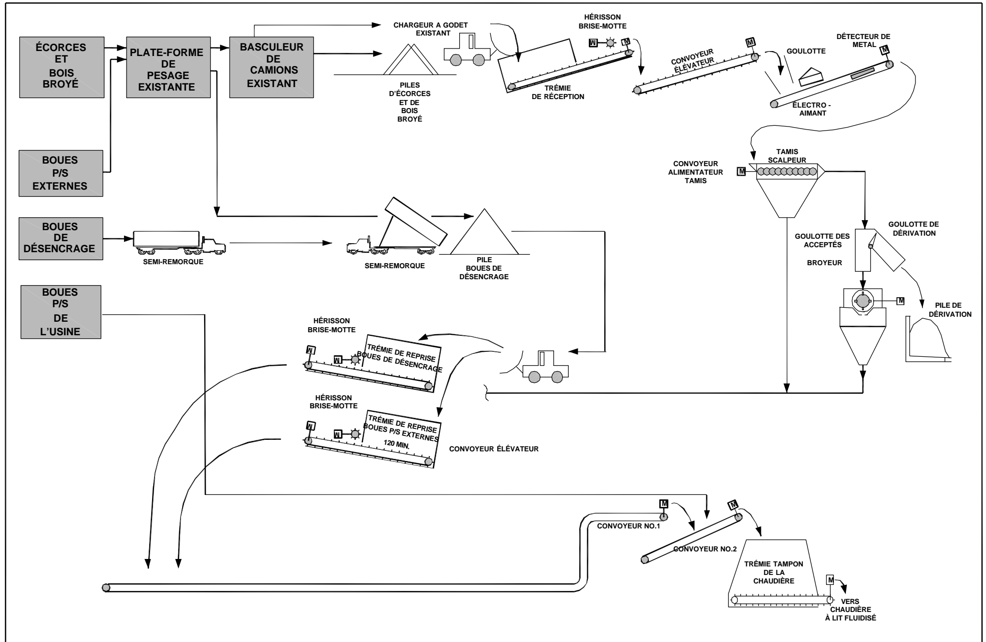
Figure 8. Système de manutention de la biomasse
