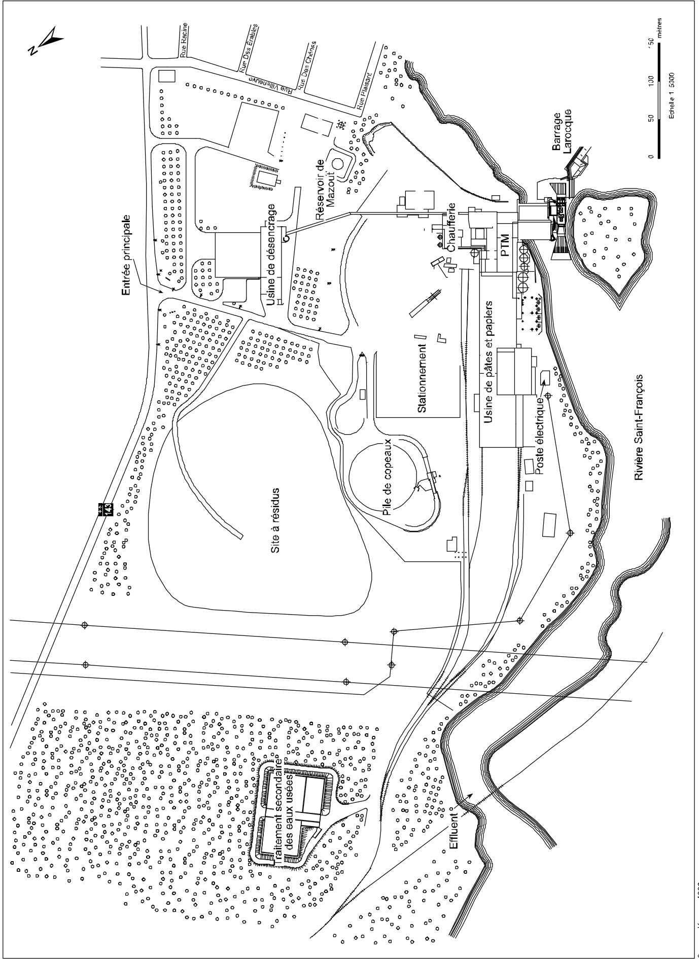
Figure 2. Installations actuelles de l'usine Kruger Brompton
