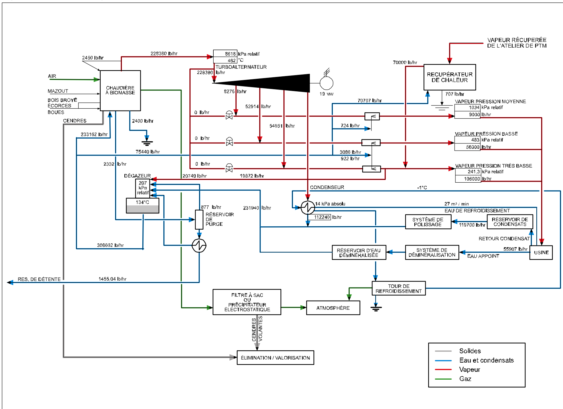
Figure 14. Schéma de procédé et bilan - conditions d'été
