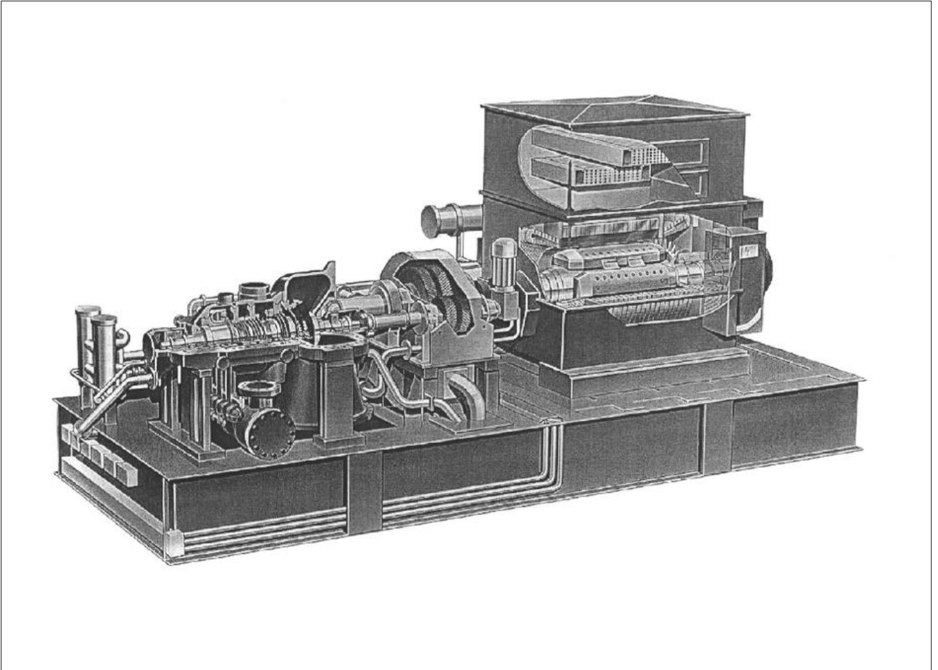
Figure 13. Croquis d'un turboalternateur
